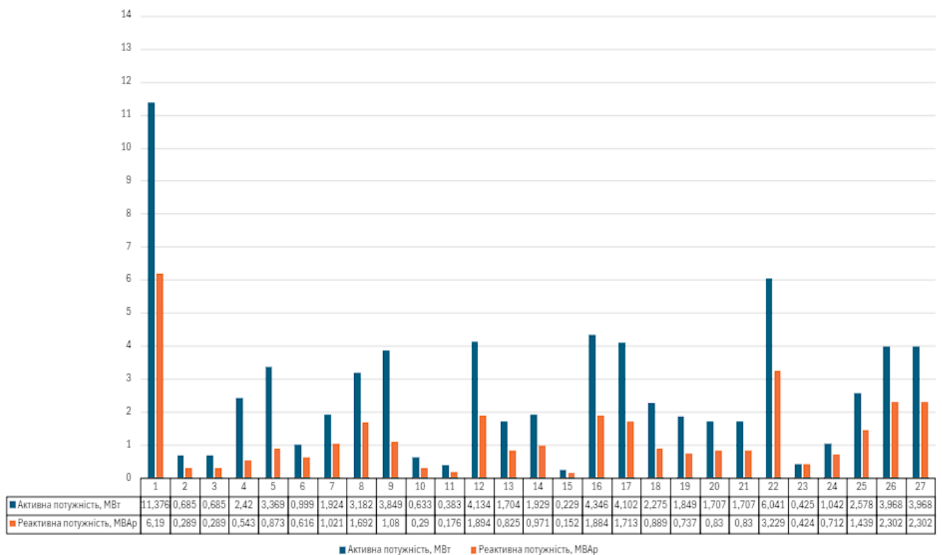
Рисунок 2.14 – Результати розрахунку перетоків по ділянкам усталений режим роботи ЕМ (літній мінімум)
