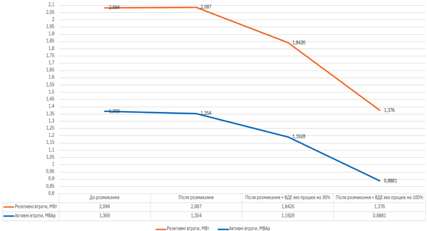
Рисунок 3.17 – Графік активних та реактивних втрат в ЛЕП ЕМ при зимовому максимумі та різних режимах роботи
