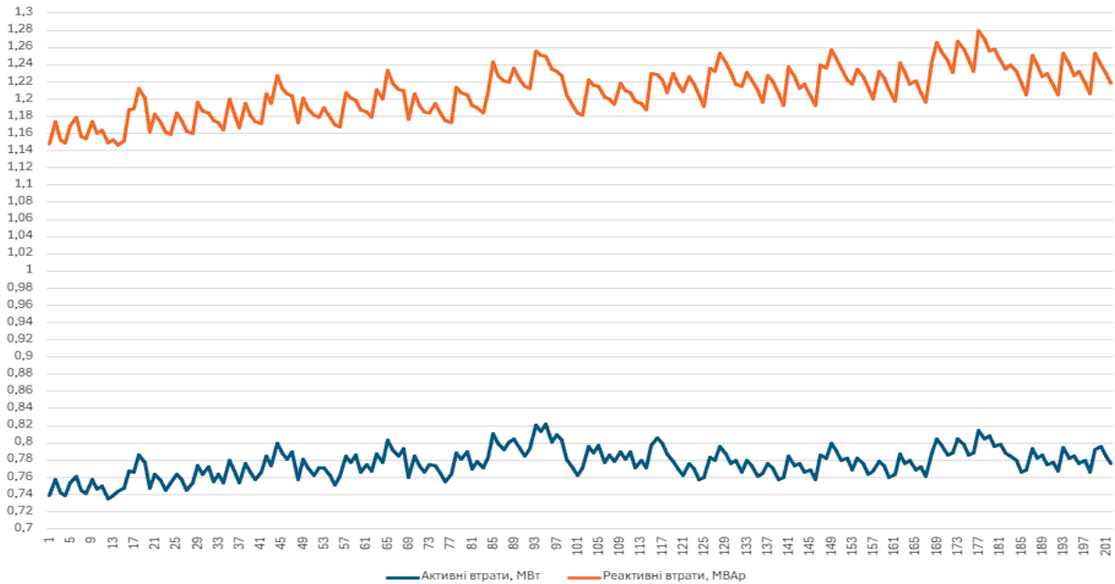
Рисунок 4.1 – Сумарні активні та реактивні втрати в ЛЕП відповідно варіанту моделювання (вісь X – відповідність даних про втрати № варіанту в табл. Б.1)
