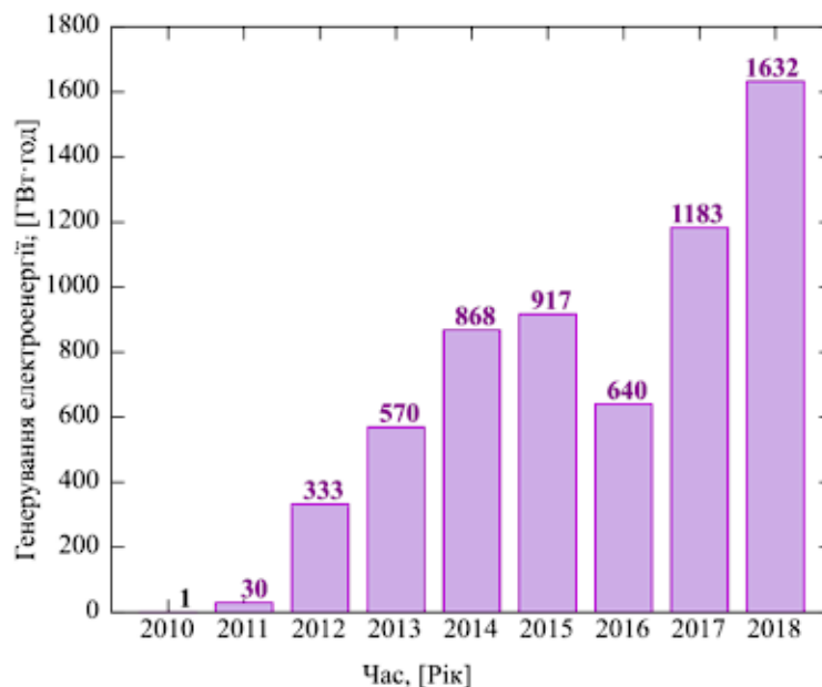
Рисунок 3.1 - Тенденція збільшення генерування електроенергії ФЕС в Україні за даними IRENA
