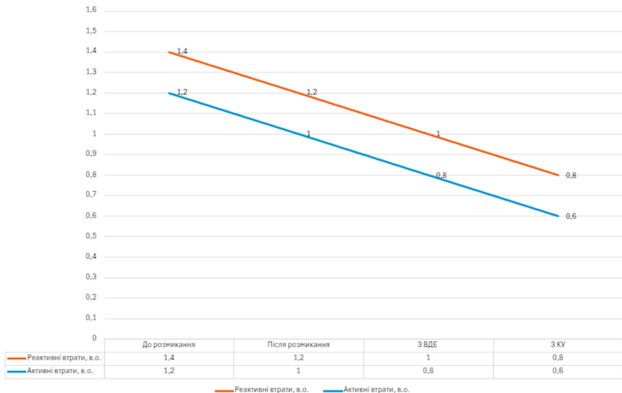
Рисунок 5.1 – Поетапне зниження активних та реактивних втрат в в.о. при застосуванні вдосконаленої методики підвищення енергоефективності ЕМ
