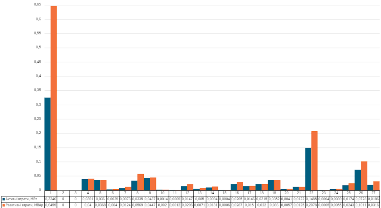
Рисунок 3.12 – Результати розрахунку втрат по ділянках усталений режим роботи ЕМ (зимовий максимум) після розмикання (відключення лінії Пісочин – Люботин) з ВДЕ
