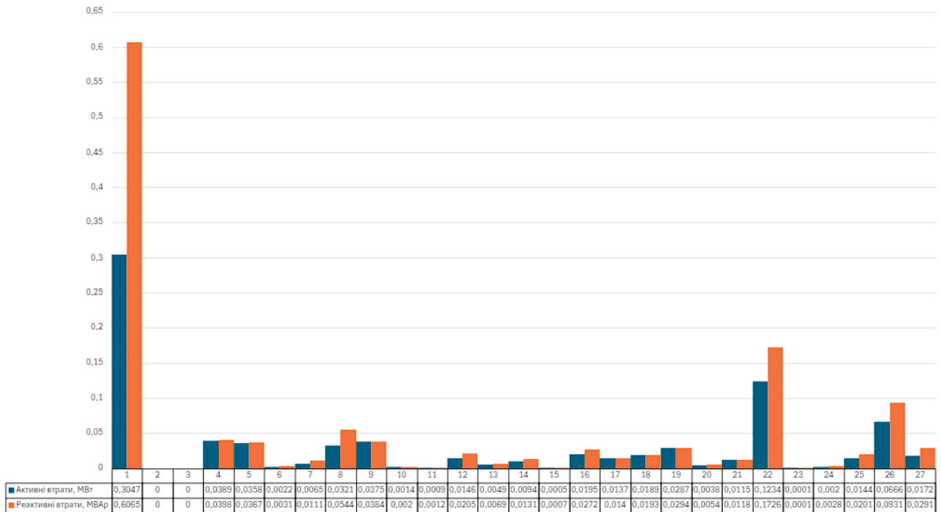
Рисунок 3.20 – Результати розрахунку втрат по ділянкам усталений режим роботи ЕМ (зимовий максимум) після розмикання (відключення лінії Пісочин – Люботин) при роботі ВДЕ з \cos\varphi = 0,9
