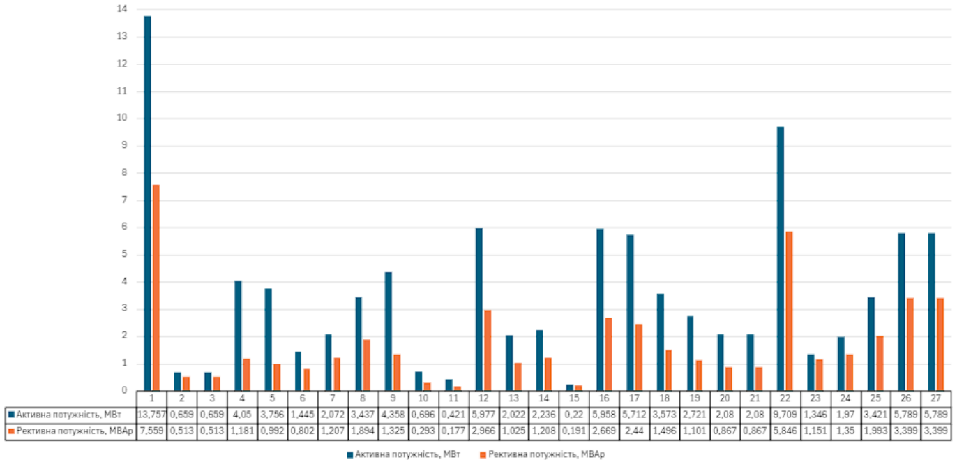
Рисунок 2.8 – Результати розрахунку усталеного режиму ЕМ (зимній максимум) перетоки по ділянках (вісь X – номери ділянок ЕМ, згідно табл. 2.4, вісь Y – МВт/МВАр)
