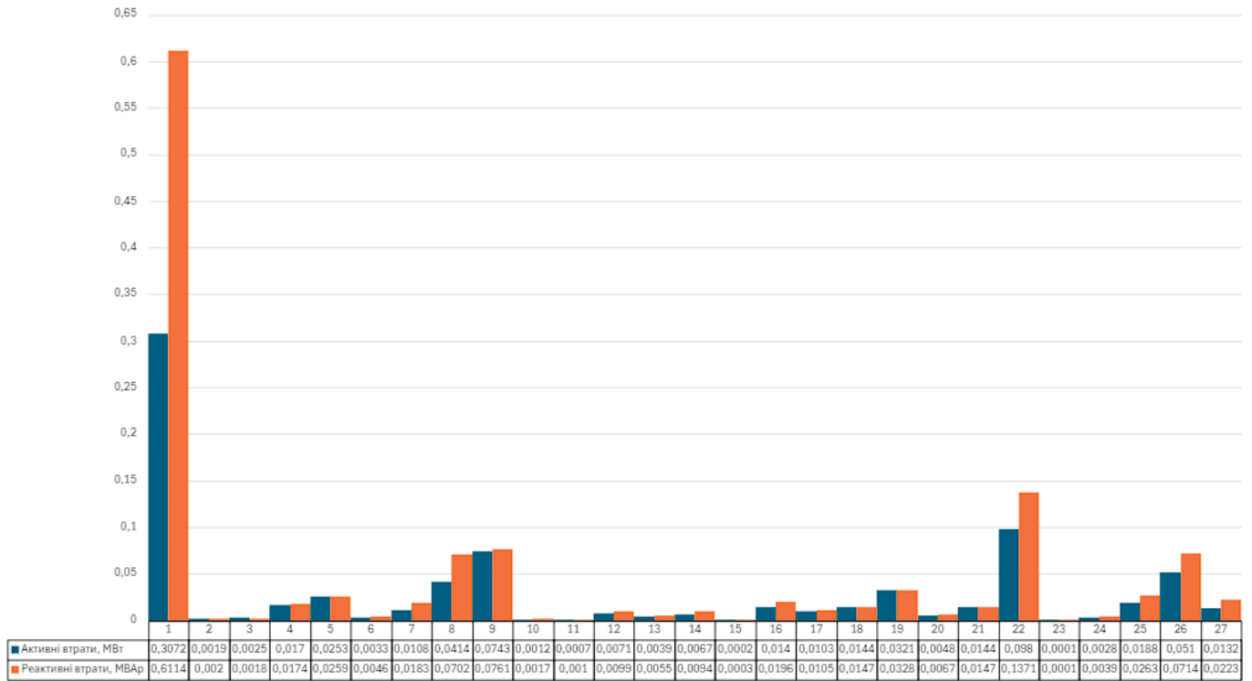
Рисунок 2.15 – Результати розрахунку втрат по ділянкам усталений режим роботи ЕМ (літній мінімум)
