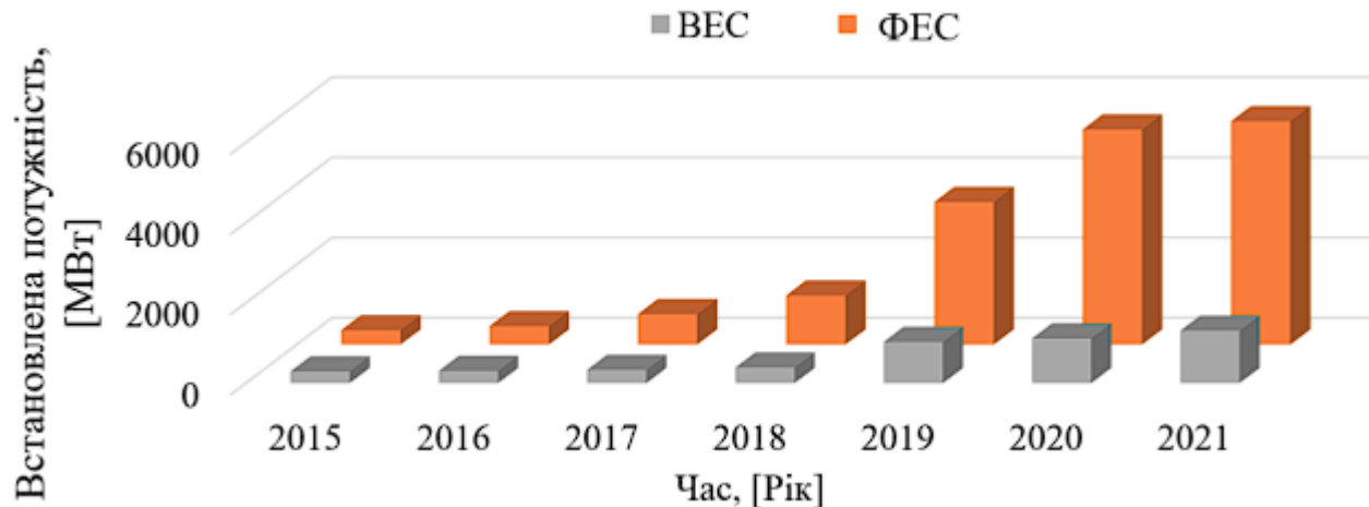
Рисунок 3.2 - Встановлена потужність ВДЕ в Україні за даними НЕК «Укренерго»
