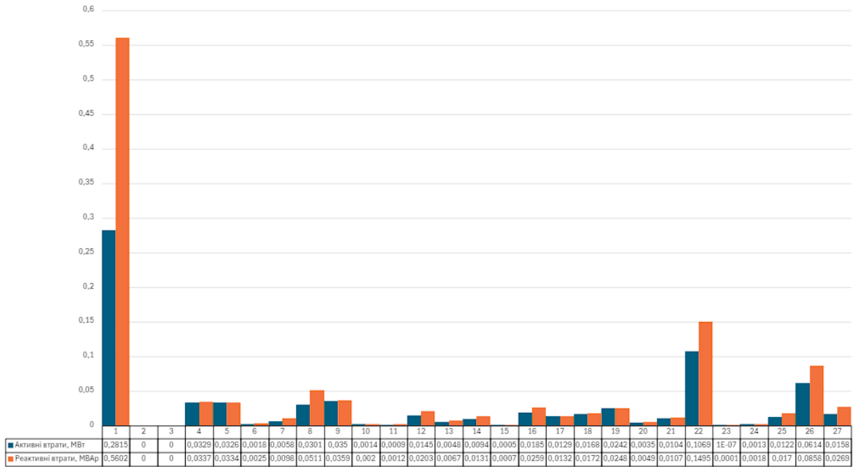
Рисунок 4.4 – Результати розрахунку втрат по ділянкам усталений режим роботи ЕМ (зимовий максимум) після розмикання, з ВДЕ при \cos\phi = 1 та з 4 КУ
