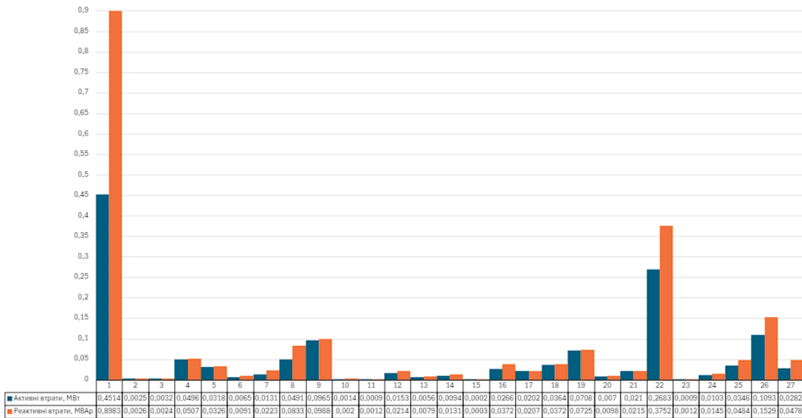
Рисунок 2.9 – Результати розрахунку усталеного режиму ЕМ (зимній максимум) втрати потужності по ділянках (вісь X – номери ділянок ЕМ, згідно табл. 2.4, вісь Y – МВт/МВАр)
