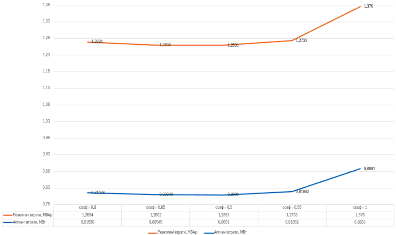
Рисунок 3.18 – Залежність втрат в ЛЕП від різних значень \cos\phi ВДЕ (СЕС)
