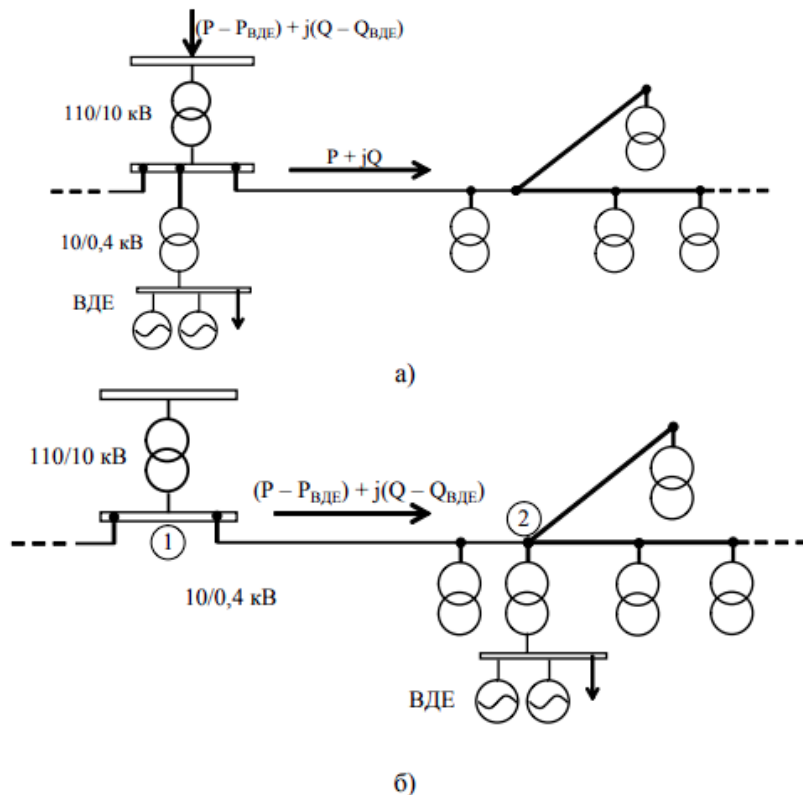
Рисунок 3.4 - Варіанти підключення ВДЕ до ЕМ
