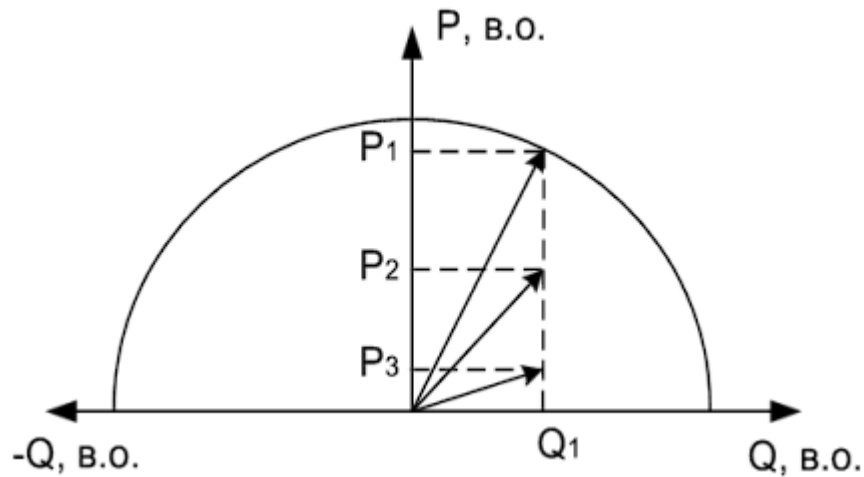
Рисунок 3.7 – Характеристика потужності ВДЕ з фіксованим значенням реактивної потужності
