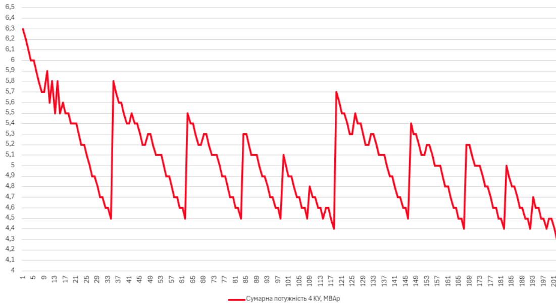
Рисунок 4.2 – Сумарна потужність 4 КУ відповідно варіанту моделювання (вісь X – відповідність даних про втрати № варіанту в табл. Б.1)
