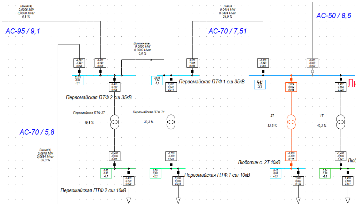
Рисунок 2.5 – Видягд ПС 35/10кВ в PowerFactory
