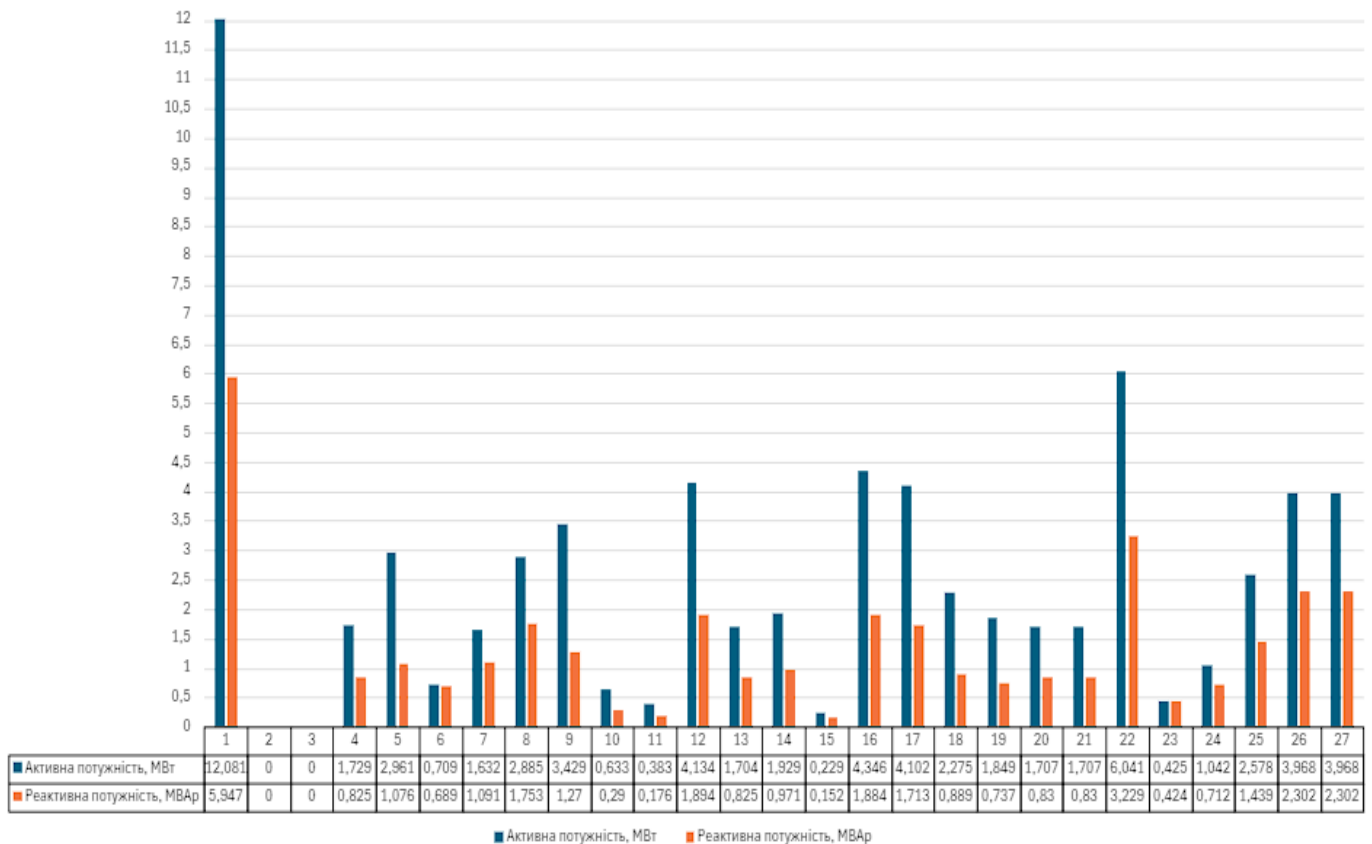
Рисунок 2.17 – Результати розрахунку перетоків по ділянкам усталений режим роботи ЕМ (літній мінімум) при відключенні лінії Пісочин – Люботин
