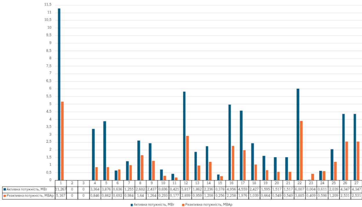
Рисунок 4.3 – Результати розрахунку перетоків по ділянкам усталений режим роботи ЕМ (зимовий максимум) після розмикання, з ВДЕ при \cos\phi = 1 та з 4 КУ
