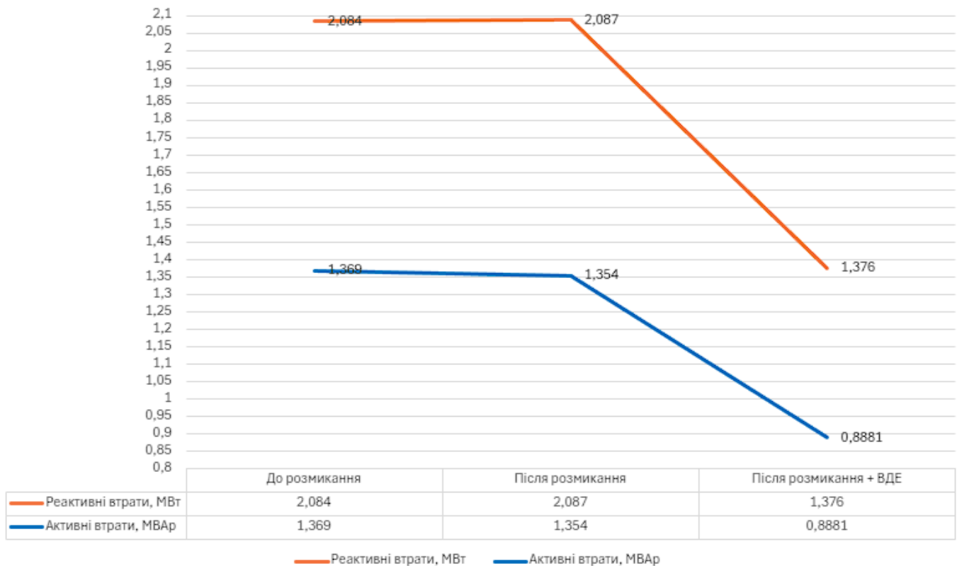
Рисунок 3.14 – Графік активних та реактивних втрат в ЛЕП ЕМ при зимовому максимумі та різних режимах роботи
