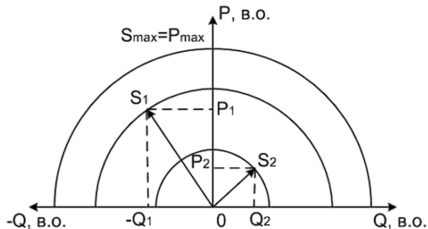
Рисунок 3.8 – Характеристика потужності ВДЕ в режимі регулювання напруги
