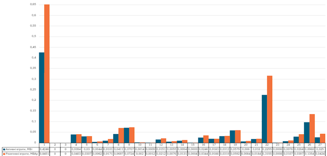
Рисунок 3.16 – Результати розрахунку втрат по ділянках усталений режим роботи ЕМ (зимовий максимум) після розмикання (відключення лінії Пісочин – Люботин) з ВДЕ яке працює на 30%
