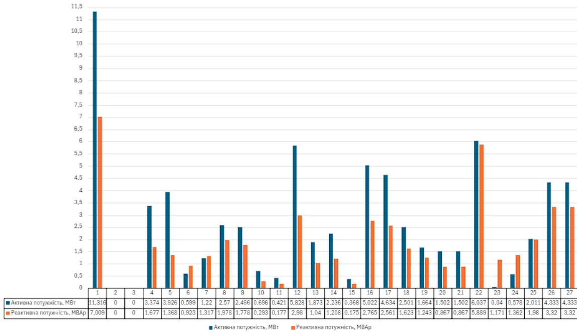
Рисунок 3.11 – Результати розрахунку перетоків по ділянках усталений режим роботи ЕМ (зимовий максимум) після розмикання (відключення лінії Пісочин – Люботин) з ВДЕ
