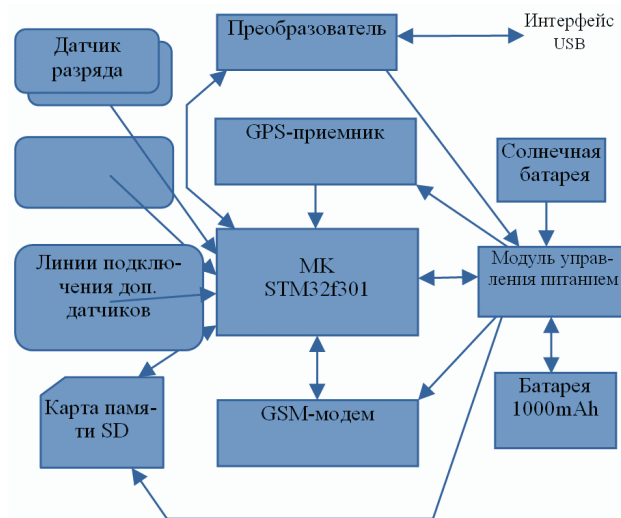
Рисунок 2 – Общая схема автономного модуля
