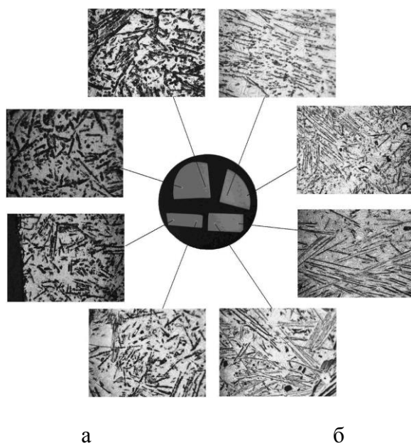
Рис. 8 – Металографічне дослідження зразка: а – зразок без обробки; б – зразок після обробки ГУП
