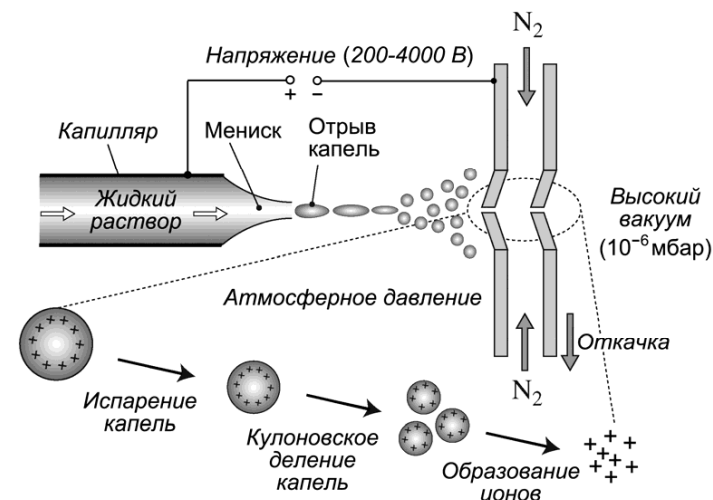
Рисунок 67 – Схема электроспрей-ионизации ESI
