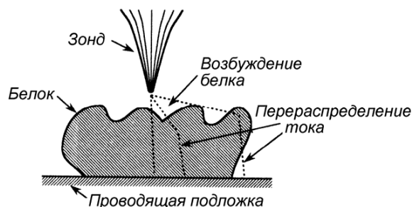
Рисунок 64 – Факторы, снижающие разрешение СТМ биологических объектов
