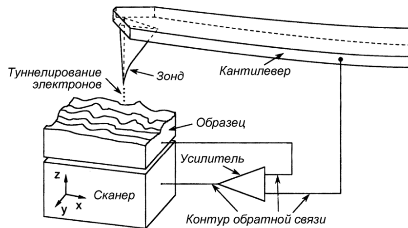
Рисунок 60 – Схема сканирующего туннельного микроскопа
