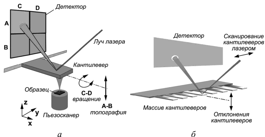
Рисунок 82 – Схема массива кантилеверов: а – движения кантилевера в атомно-силовом микроскопе; б – лазерное считывание кантилеверов
