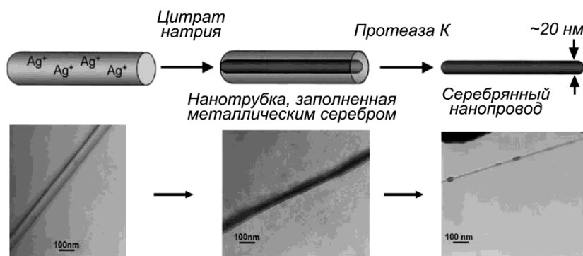
Рисунок 231 – Синтез серебряных нанопроводов с помощью ADPN
