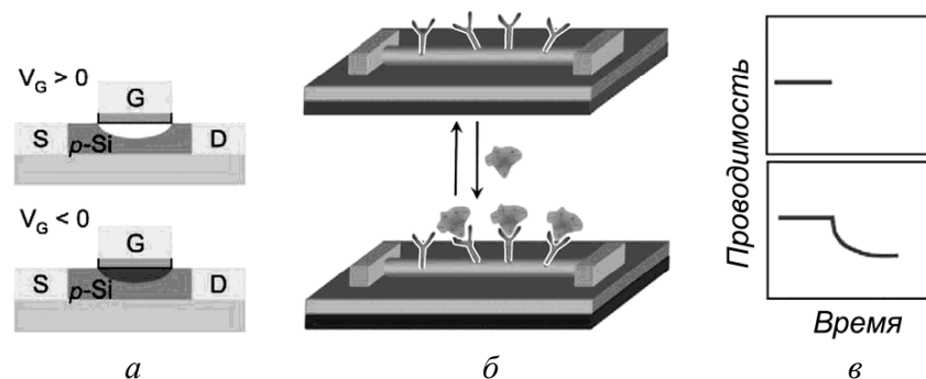
Рисунок 247 – Нанопроводной FET-сенсор: а – режимы работы полевого p -Si транзистора; б – схема Si-нанопроводникового FET-сенсора, сенсibilизированного антителами в качестве рецепторов анализитов; в – изменение проводимости сенсора при связывании с положительно заряженным белком
