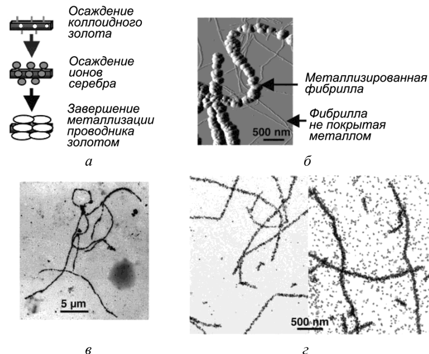
Рисунок 228 – Металлизация прионовых нанофибрилл: а – этапы металлизации; б – АСМ-изображение; в – ТЕМ-изображение; г – влияние режимов металлизации на диаметр нанопроводников
