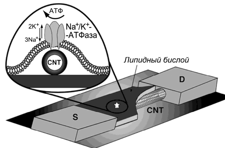
Рисунок 249 – Схема FET-CNT-транзистора
