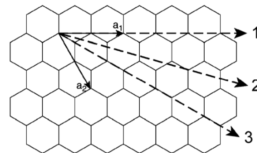
Рисунок 94 – Варианты сворачивания графенового листа в углеродную нанотрубку: 1 – "зигзаг"; 2 – хиральная трубка; 3 – "кресло"
