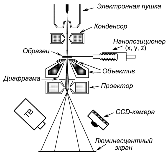
Рисунок 52 – Схема просвечивающего электронного микроскопа
