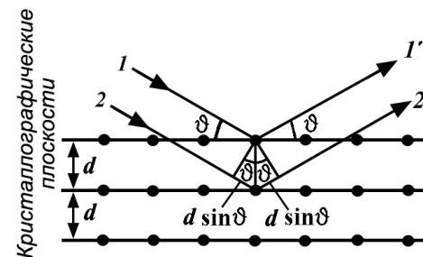
Рисунок 36 – Дифракция на кристаллической решетке
