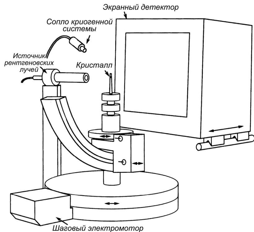
Рисунок 37 – Схема рентгеновского дифрактометра
