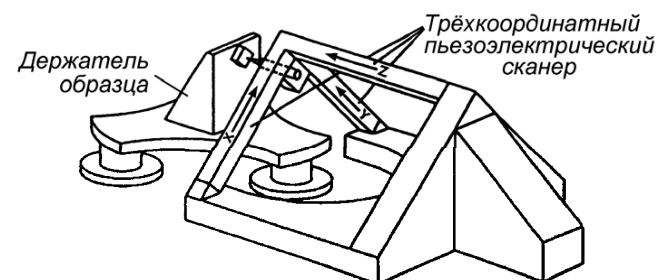
Рисунок 63 – Сканирующий механизм туннельного микроскопа
