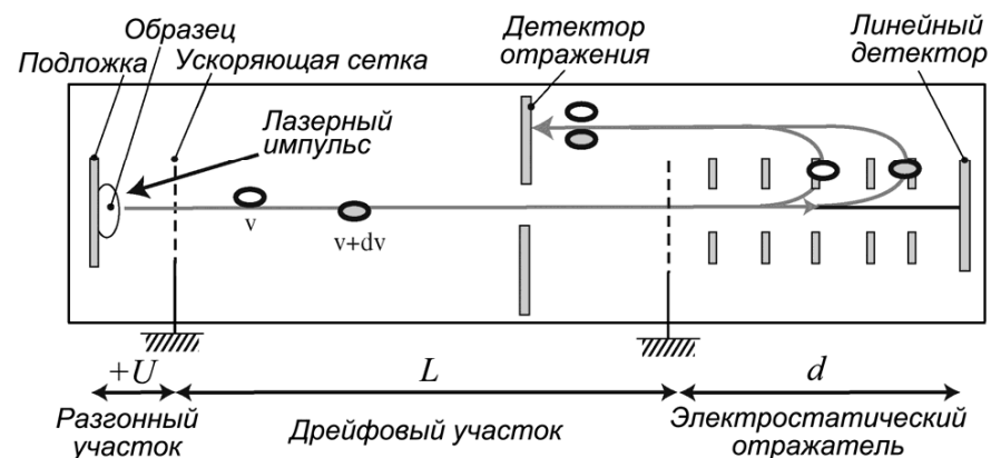
Рисунок 76 – Схема отражательного время-пролётного масс-спектрометра
