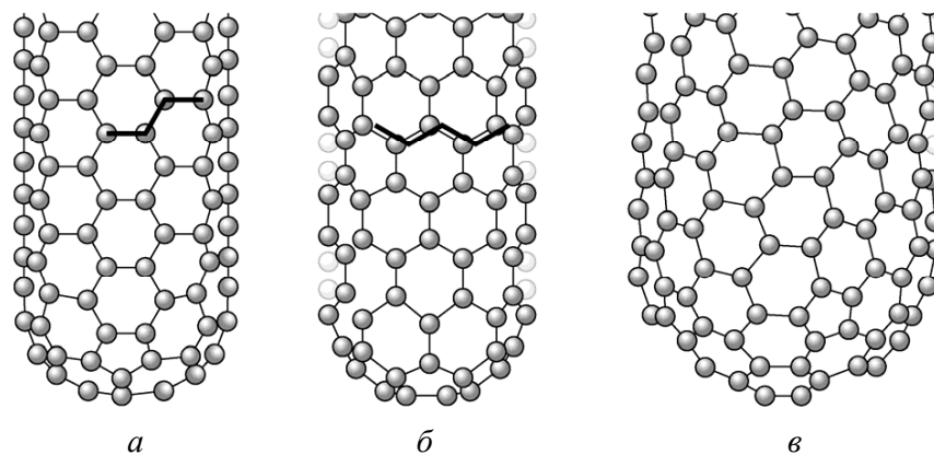
Рисунок 95 – Нанотрубки различной хиральности: a – нанотрубка типа "кресло"; б – нанотрубка типа "зигзаг"; в – хиральная нанотрубка
