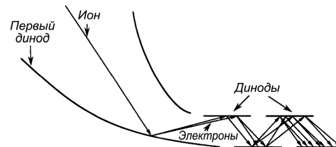
Рисунок 79 – Схема ВЭУ
