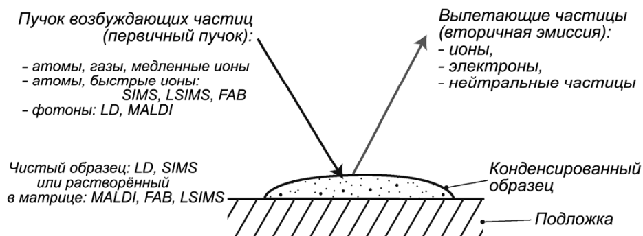
Рисунок 66 – Схема ионизации твердого образца
