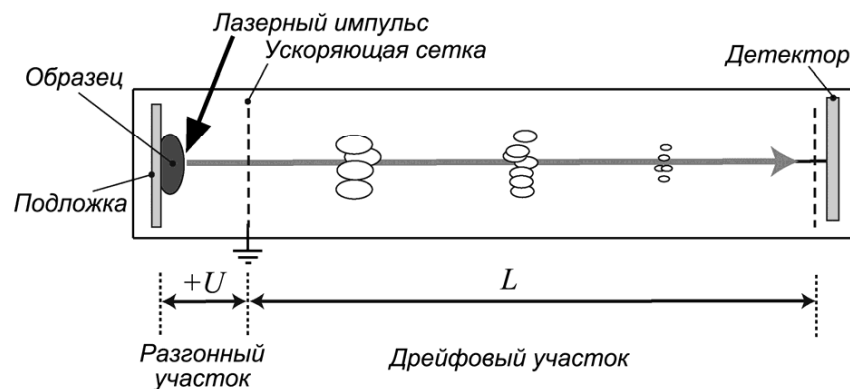
Рисунок 75 – Схема линейного время-пролётного масс-спектрометра
