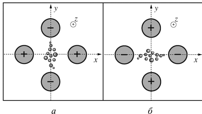
Рисунок 73 – Осцилляции ионного пучка в квадрупольном анализаторе: а – к концу первой половины периода осцилляции; б – к концу второй половины периода
