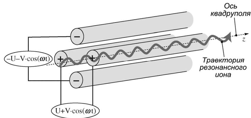
Рисунок 72 – Схема квадрупольного анализатора масс
