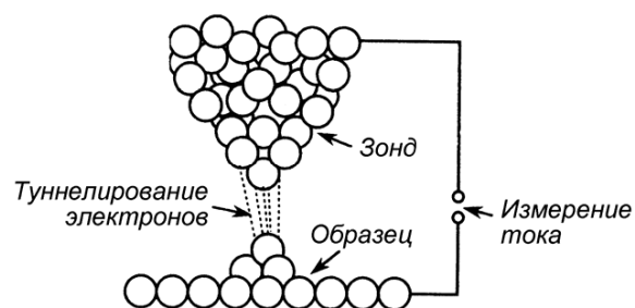
Рисунок 61 – Взаимодействие зонда с поверхностью образца
