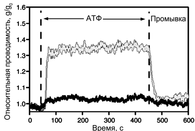
Рисунок 250 – Изменение проводимости FET-CNT-транзистора
