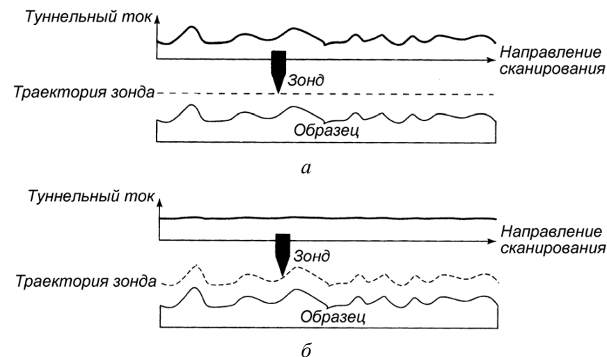
Рисунок 62 – Режимы сканирования СТМ: а – постоянной высоты зонда; б – постоянного тока
