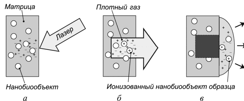
Рисунок 69 – Схема лазерно-десорбционной ионизации с участием конденсированной матрицы MALDI
