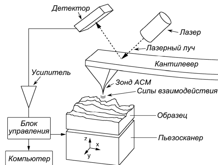
Рисунок 54 – Схема атомно-силового микроскопа (АСМ)
