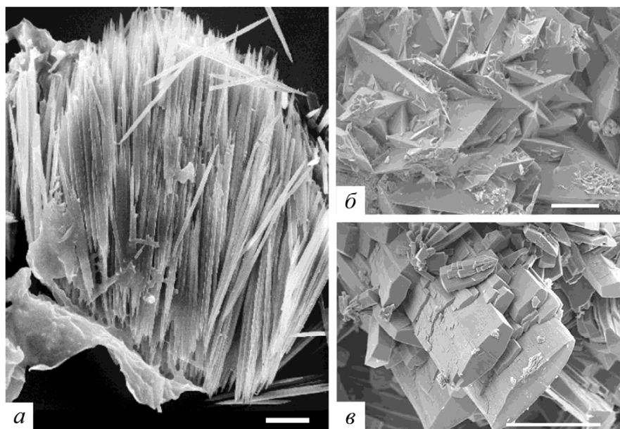
Рисунок 192 – Примеры биоминерализации
