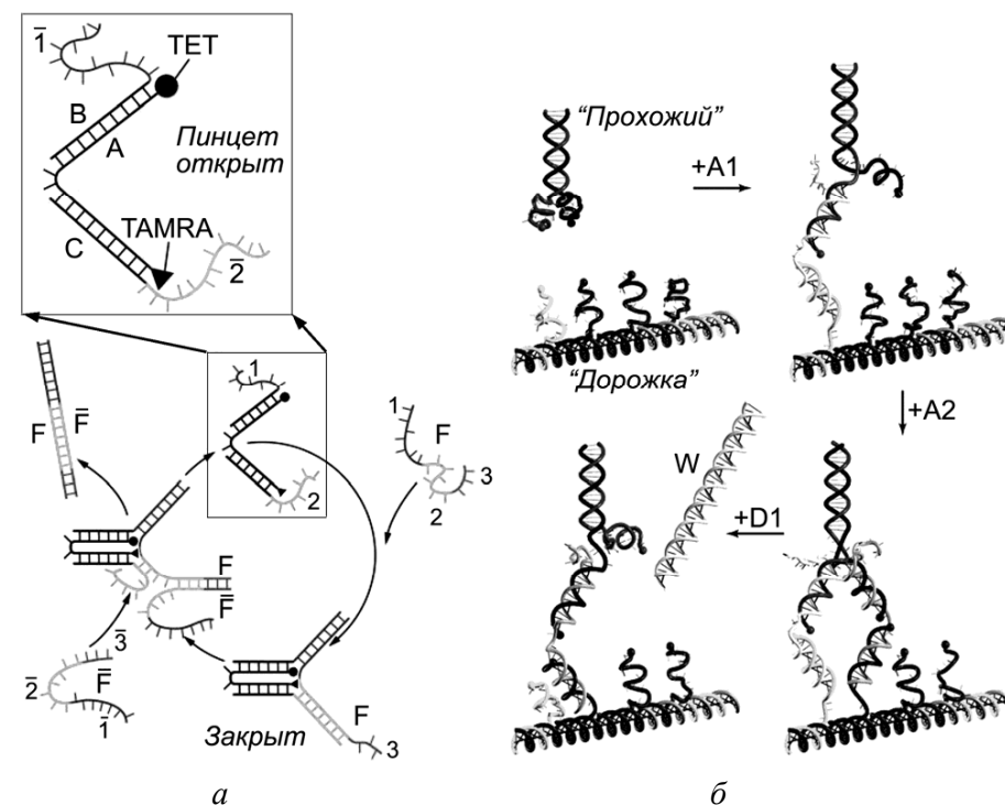
Рисунок 260 – ДНК-механизмы: а – схема ДНК-пинцета; б – шагающая ДНК
