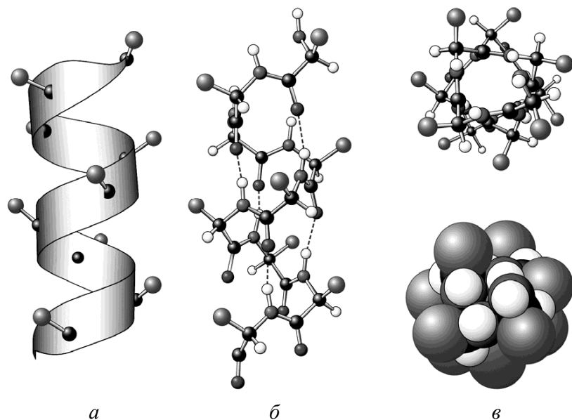
Рисунок 122 – Белковая \alpha -спираль: а – изображение в виде "резиновой ленты", б – схема связей, вид сбоку, в – проекция вдоль оси спирали
