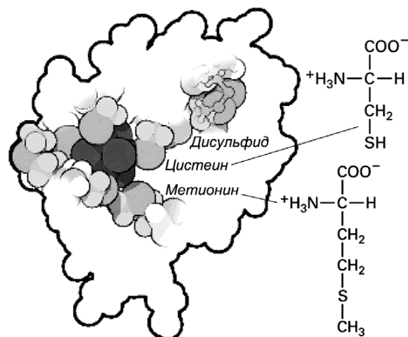
Рисунок 14 – Структурные особенности цистеина и метионина
