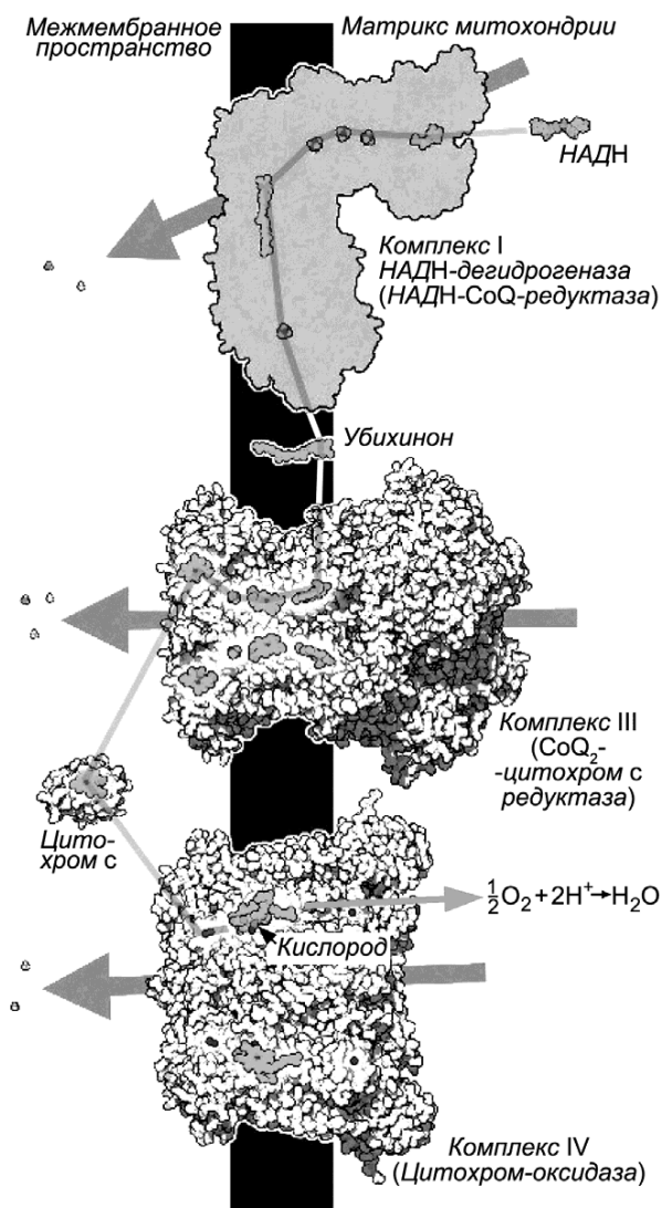
Рисунок 166 – Бионанозлектрическая цепь сопряжения электронного транспорта с созданием протонного градиента (дыхательная цепь)
