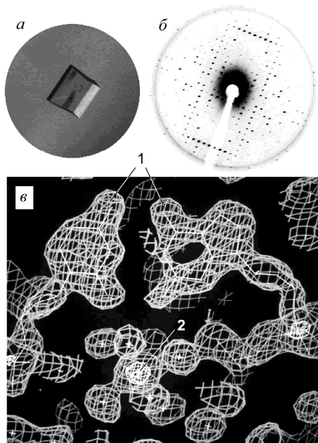
Рисунок 43 – Рентгеновская кристаллография: а – кристалл из биомолекул; б – дифрактограмма; в – распределение плотности, восстановленное компьютером. 1 – цитозин-гуаниновая пара оснований в ДНК; 2 – ион кальция
