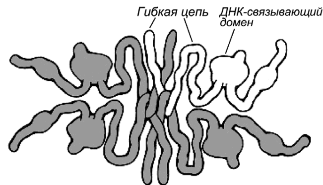
Рисунок 128 – Схема ДНК-связывающего белка p53
