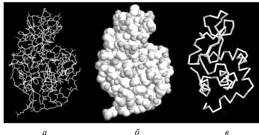
Рисунок 102 – Визуализация молекулярной структуры лизоцима: а – схема ковалентных связей; б – ван-дер-ваальсовая модель молекулы; в – "резиновая лента"
