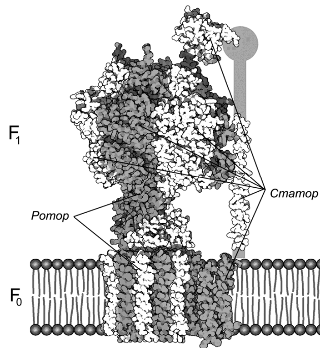
Рисунок 21 – Схема АТФ-синтазы: 1 – ротор; 2 – статор
