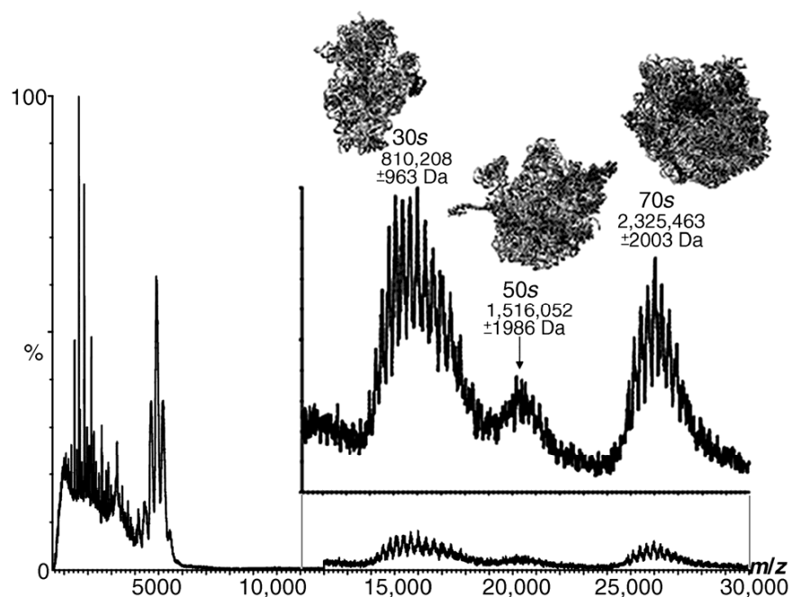
Рисунок 68 – ESI масс-спектр рибосомы Thermus thermophilus . Кроме собственно рибосомы 70S, в спектре присутствуют также серии пиков, относящихся к большой 50S и малой 30S субъединицам рибосомы
