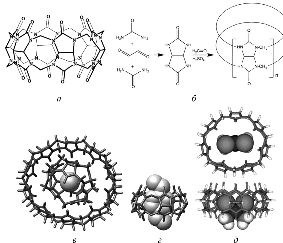
Рисунок 238 – Кукурбитурилы: а – схема кукурбит[6]урилы; б – схема синтеза; в – комплекс CB[10]•CB[5]•Cl - ; г – комплекс CB[6]• p -силилендиаммоний-хлорид; д – комплекс CB[7]•цисплатин ( cisplatin )
