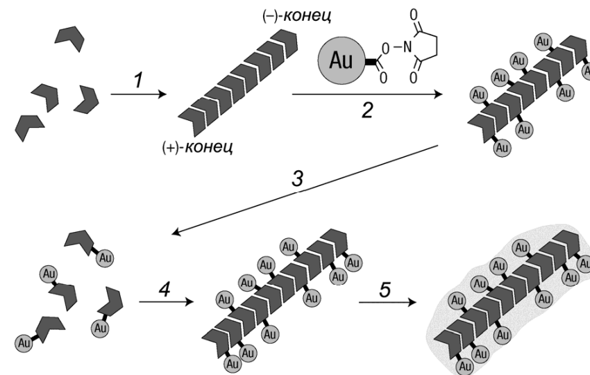
Рисунок 230 – Металлизация актиновых фибрилл
