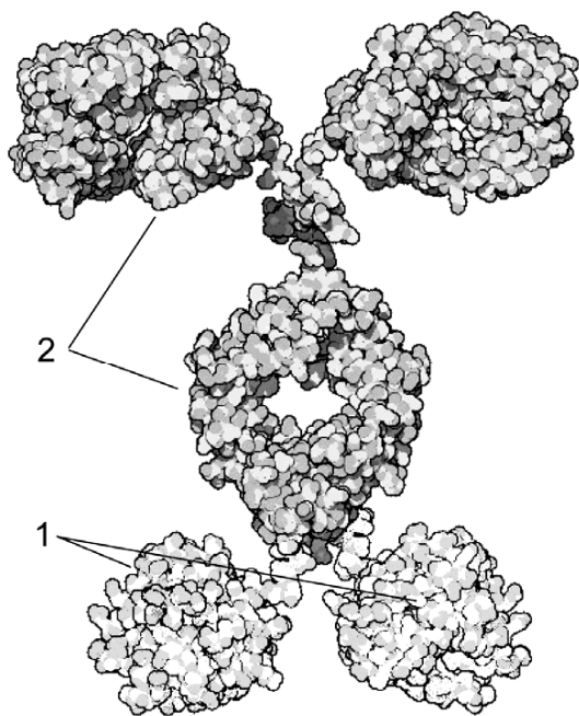
Рисунок 34 – Схема антиракового иммунотоксина: 1 – токсичный белок; 2 – антитело
