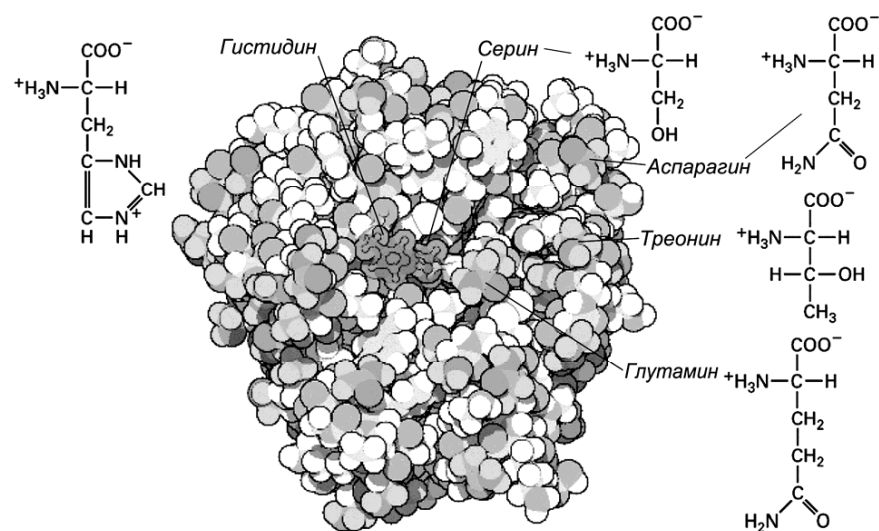
Рисунок 9 – Структурные особенности гистидина, серина, аспарагина, треонина и глутамина
