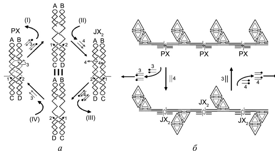
Рисунок 259 – ДНК-мотор: а – схема ДНК-реле; б – переключение ДНК-структуры
