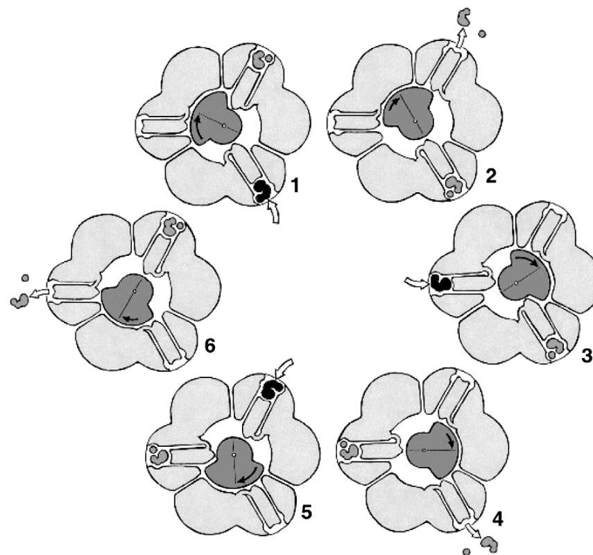
Рисунок 203 – Рабочий цикл F_1 мотора
