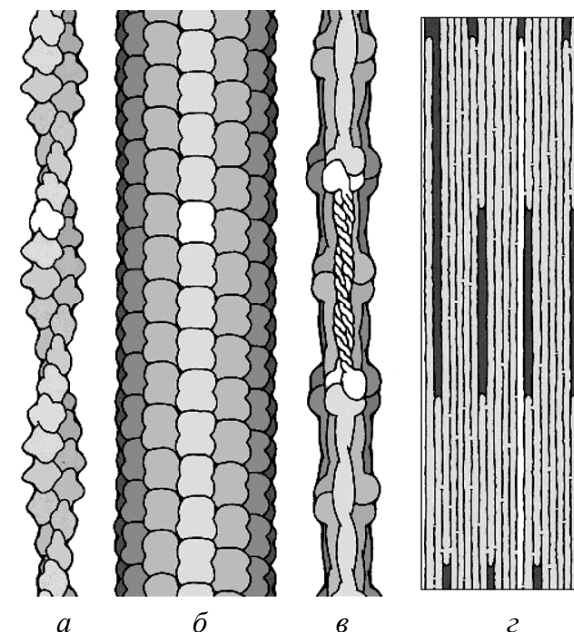
Рисунок 177 – Модульные филаменты: а – актиновая нить, б – микротрубочка, в – промежуточный филамент, г – коллаген
