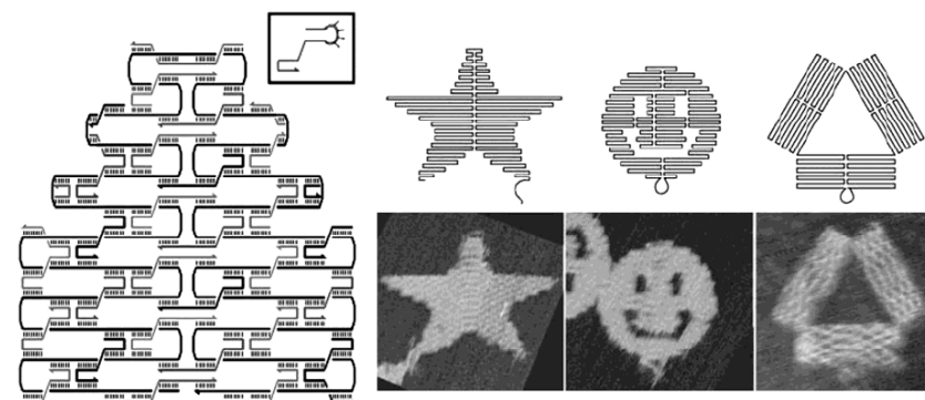
Рисунок 253 – ДНК-оригами: схема укладки элементов (слева) и синтезированные ДНК-изображения (справа)
