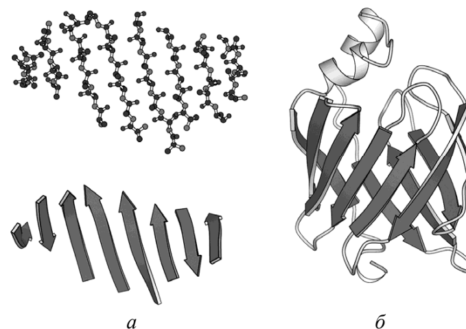
Рисунок 121 – \beta -Структуры: а – разные способы наглядного представления (визуализации), б – третичная структура собранная из \beta -структур
