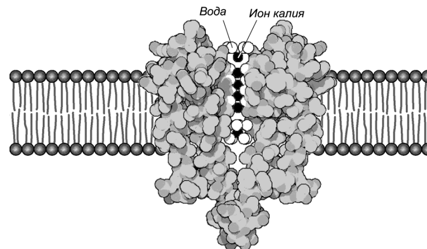
Рисунок 209 – Схема калиевого канала биомембраны
