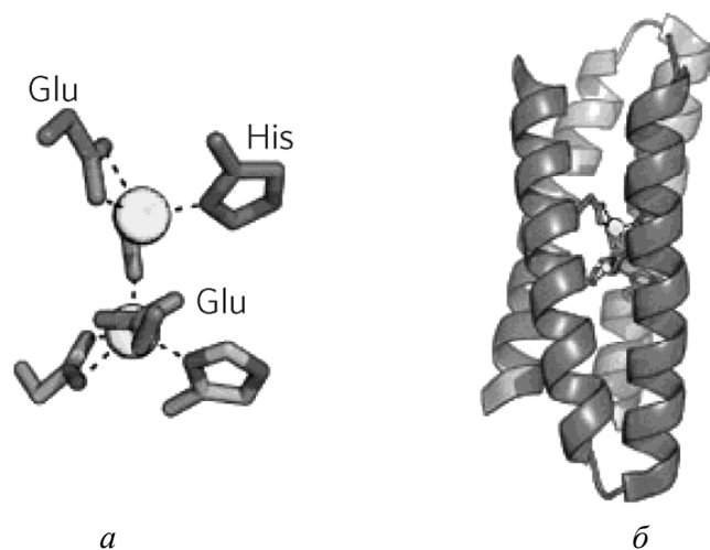
Рисунок 220 – Белок DF1: a – схема металлсвязывающего центра; б – схема упаковки полипептидной цепи белка DF1
