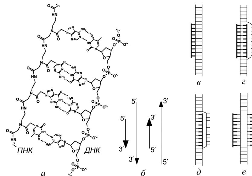
Рисунок 222 – ПНК-ДНК гибридизация: а – схема спаривания азотистых оснований; б – ориентация нитей; в – триплекс ПНК-ДНК; г – триплексная инвазия (внедрение); д – дуплексная инвазия; е – двойная дуплексная инвазия
