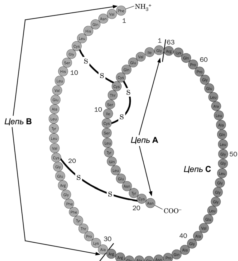
Рисунок 126 – Первичная структура проинсулина
