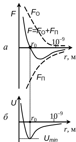
Рисунок 109 – Межмолекулярное взаимодействие: a – сила межмолекулярного взаимодействия; б – потенциальная энергия
