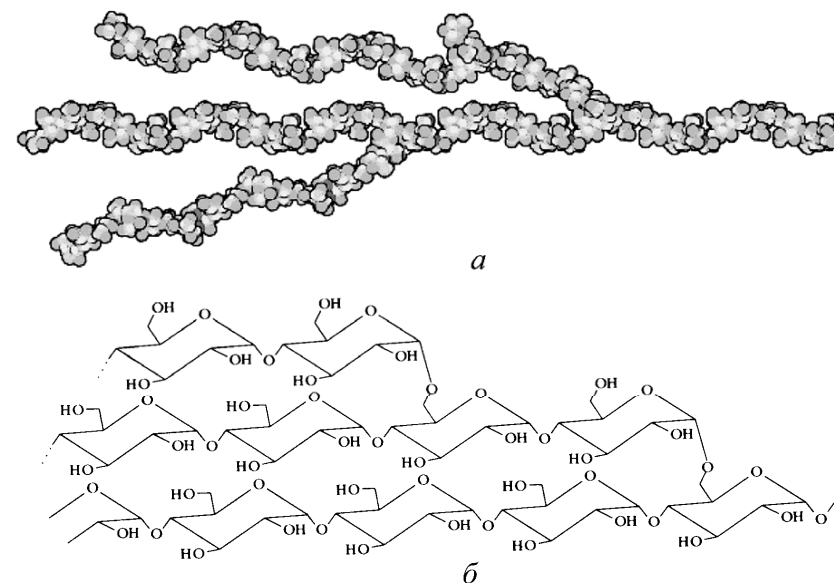
Рисунок 17 – Полисахариды: а – схема дендромерной молекулы полисахарида; б – схема связей в молекуле гликогена
