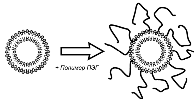
Рисунок 244 – Образование стэлс-липосомы
