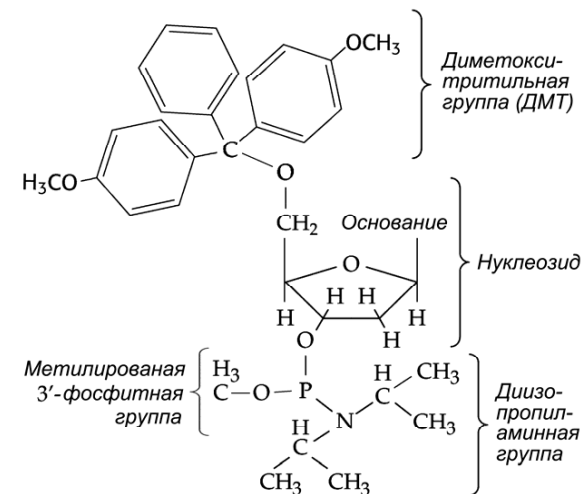
Рисунок 29 – Фосфорамидит
