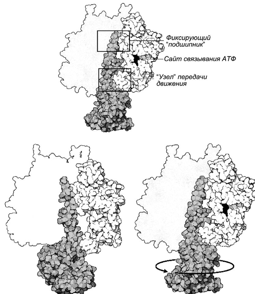
Рисунок 205 – Конформационные изменения в F_1 моторе АТФ-синтазы.
