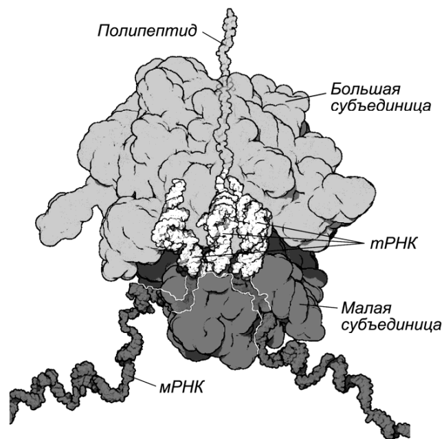
Рисунок 20 – Схема рибосомы
