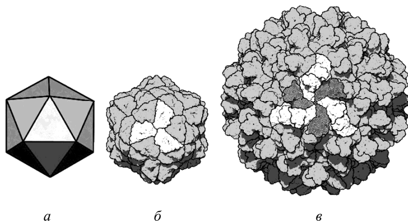
Рисунок 137 – Использование квазисимметрии при дизайне собирающихся комплексов: а – икосаэдр, б – икосаэдрический капсид малого вируса, в – икосаэдрический капсид большого вируса
