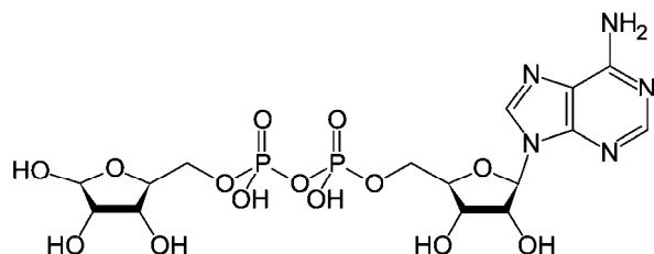
Рисунок 241 – АДФ-рибоза
