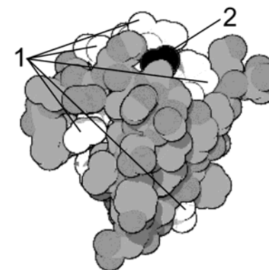
Рисунок 127 – Схема молекулы инсулина: 1 – полипептид А; 2 – дисульфидный мостик
