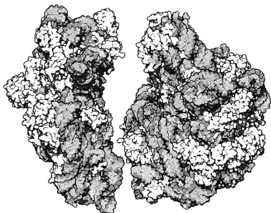
Рисунок 155 – Субъединицы рибосомы; серым цветом выделены рибосомные РНК, белым – рибосомные белки
