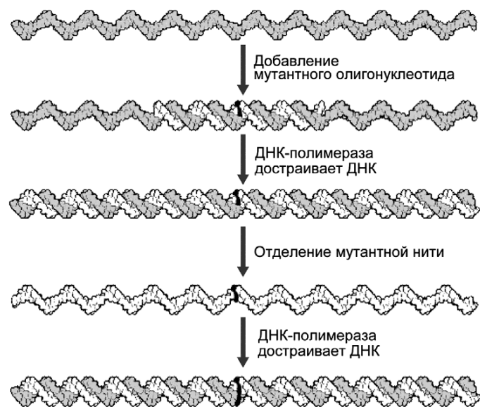
Рисунок 32 – Схема сайт-специфического мутагенеза
