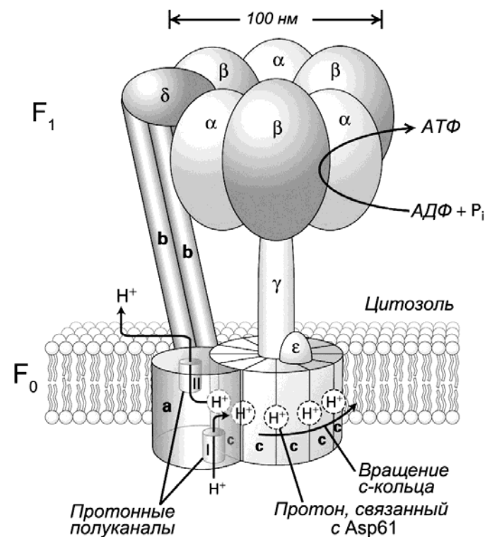
Рисунок 201 – Схема АТФ-синтазы в плазматической мембране бактерий
