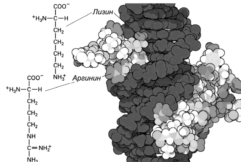
Рисунок 13 – Структурные особенности лизина и аргинина (темно-серым цветом изображена молекула ДНК)
