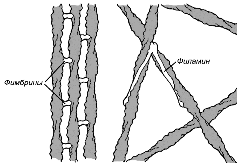
Рисунок 184 – Связывание актиновых нитей в различные инфраструктуры с помощью актин-связывающих белков, изображенных белым цветом
