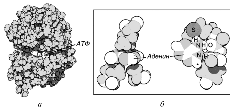
Рисунок 143 – Молекулярное распознавание аденина: а – протеин-киназа А, б – сайт связывания аденина цАМФ
