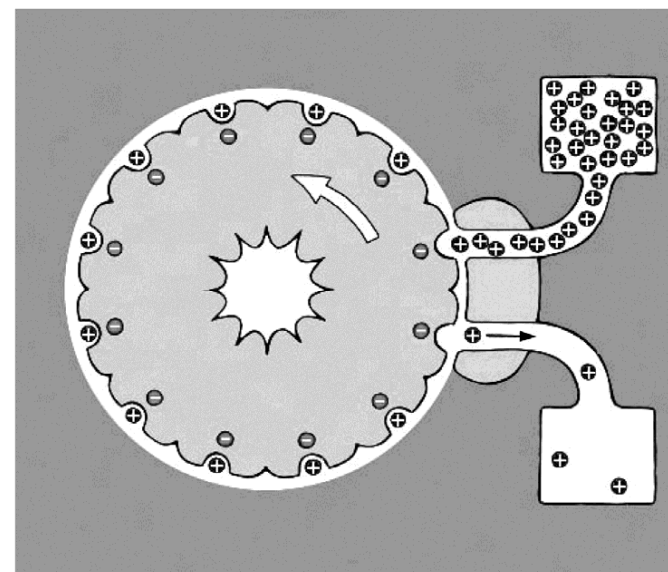
Рисунок 202 – Принцип работы ротора АТФ-синтазы
