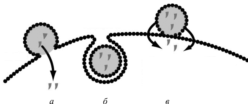
Рисунок 243 – Способы доставки лекарств в клетку липосомами: а – слияние с плазматической мембраной; б – эндоцитоз; в – облегчённая диффузия из адсорбированной липосомы
