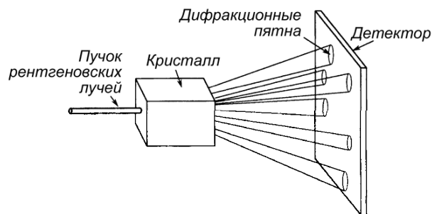
Рисунок 39 – Схема дифракции рентгеновских лучей на кристалле
