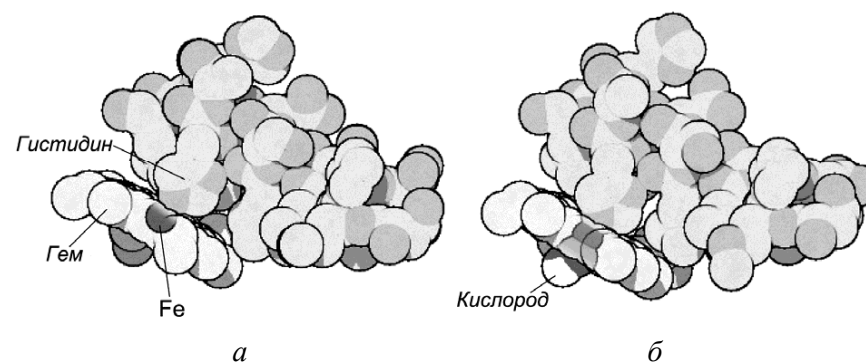
Рисунок 148 – Смещение атома железа в геме гемоглобина: а – гем без кислорода, б – гем с присоединённой молекулой кислорода
