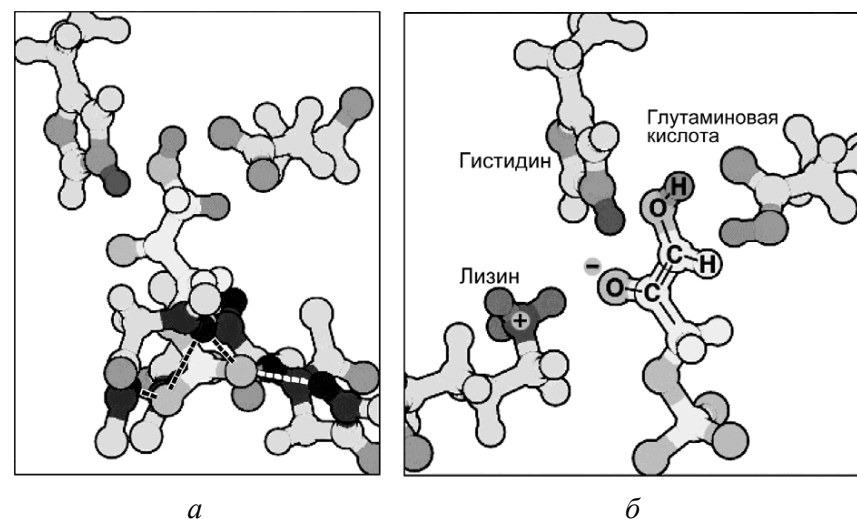
Рисунок 171 – Схемы: а – ориентации субстрата в ферменте; б – стабилизации переходного состояния
