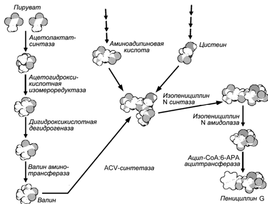
Рисунок 172 – Схема бактериального синтеза пенициллина
