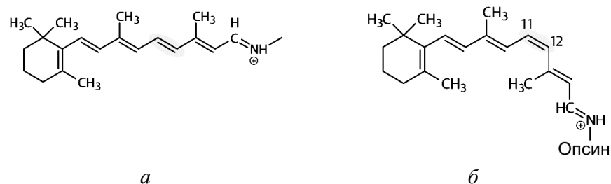
Рисунок 212 – Конформации ретиная: а – полностью- транс -ретиналь, б – 11- цис -ретиналь
