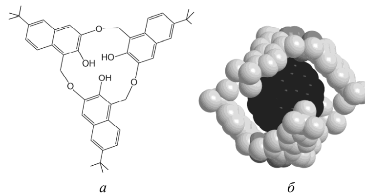
Рисунок 234 – Самосборка молекулярного наноконтейнера: а – схема гексагомо-триоксакаликс[3]трет-бутил-нафтала; б – наноконтейнер, содержащий фуллерен
