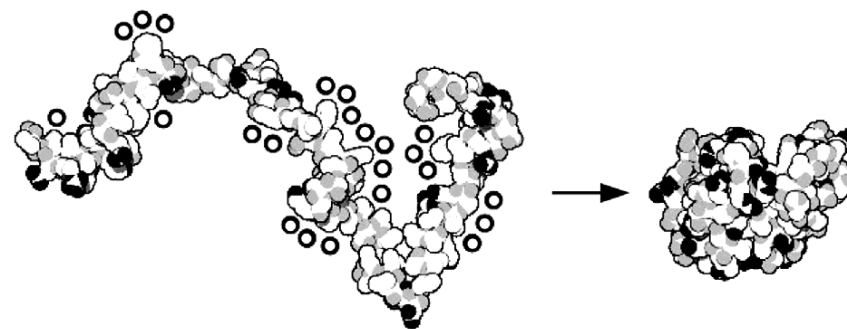
Рисунок 118 – Высвобождение молекул воды (о) при фолдинге белка лизоцим
