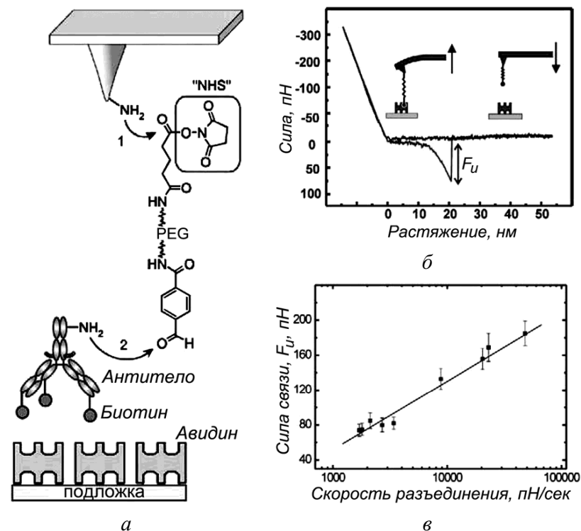
Рисунок 87 – Измерение межмолекулярных сил: а – функционализация зонда АСМ, б – определение силы связи, в – результаты измерений динамической силовой спектроскопии
