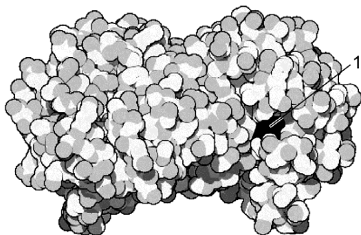
Рисунок 168 – Фермент триозофосфатизомеразы: 1 – молекула субстрата в активном центре фермента
