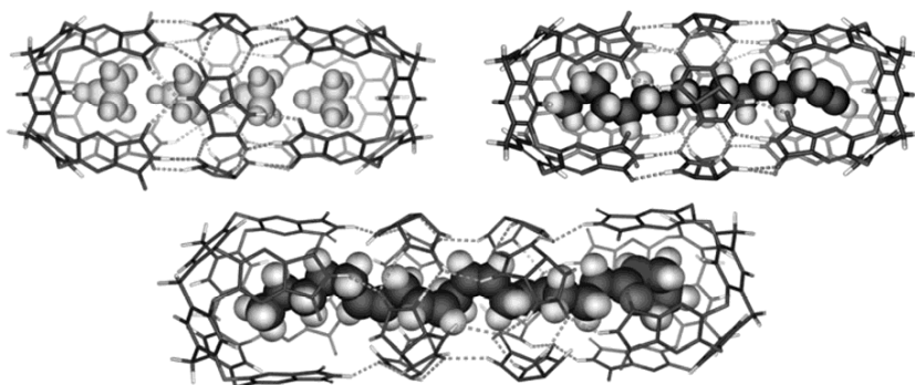
Рисунок 237 – Инкапсуляция четырёх молекул циклопропана (вверху слева), молекулы 1-гексадецена (вверху справа) и молекулы анадамида (внизу)
