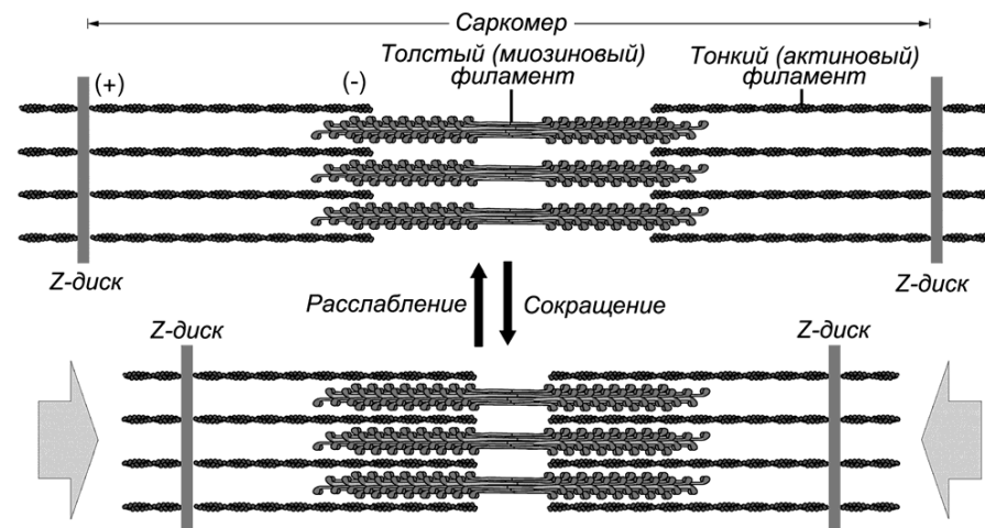
Рисунок 214 – Схема сокращения саркомера
