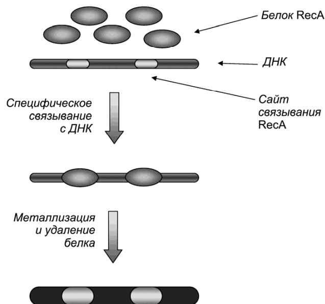
Рисунок 226 – Молекулярная литография на ДНК
