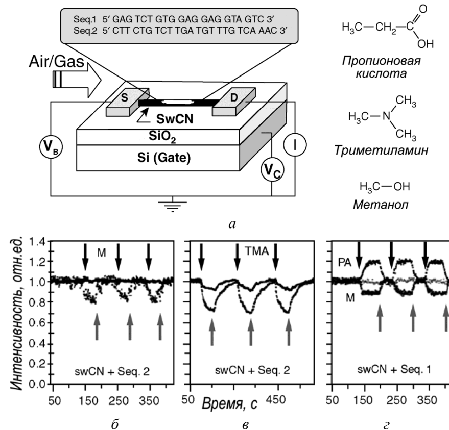
Рисунок 101 – ДНК-CNT-нанобиосенсор: а – схема сенсора и олигонуклеотидов. Детектирование молекул: б – метанола; в – триметиламина; г – метанола и пропионовой кислоты
