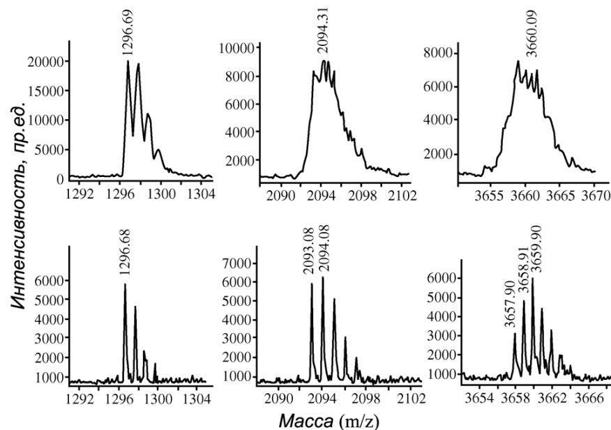
Рисунок 77 – Масс-спектры смеси пептидов записанные линейным время-пролётным масс-спектрометром (верхний ряд) и рефлектроном (нижний ряд)
