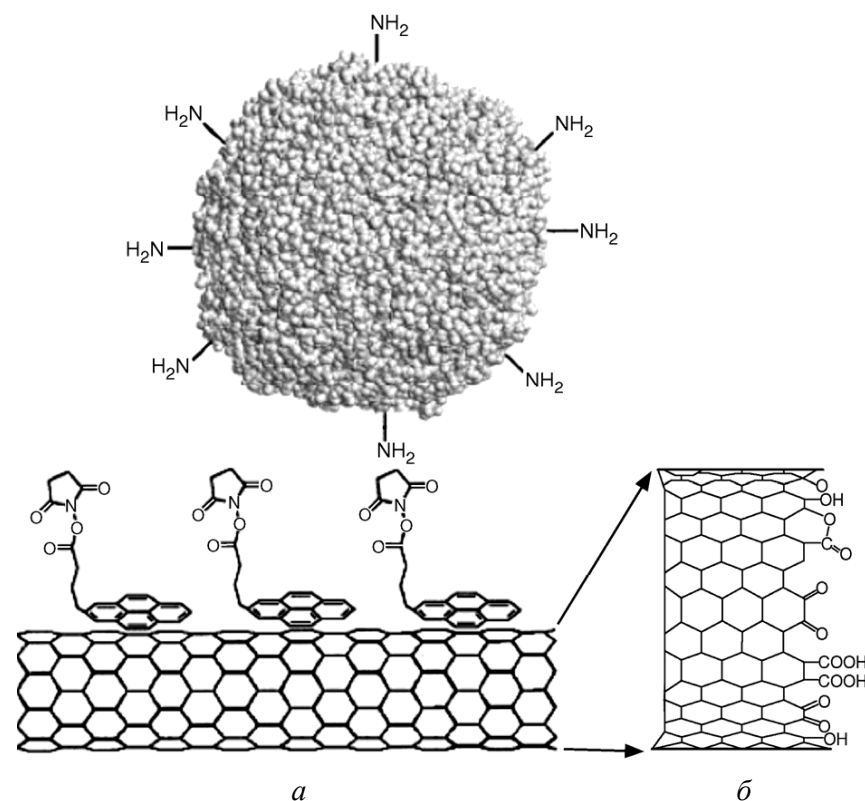
Рисунок 97 – Способы функционализации нанотрубки: а – использование нековалентно ассоциированных линкеров для функционализации нанотрубки белком; б – использование системы реакционных групп на краю нанотрубки
