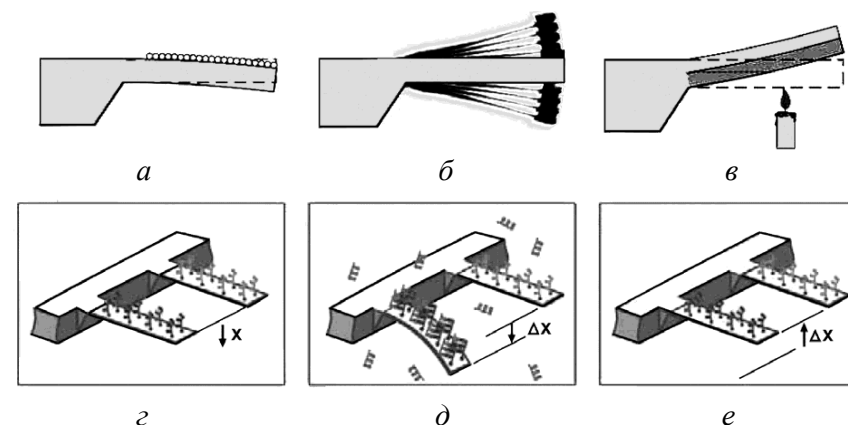
Рисунок 84 – Режимы работы сенсора: а – статический; б – динамический; в – тепловой. ДНК-гибридизационный сенсор: г – функционализация кантилеверов разными ДНК-зондами; д – смещение кантилевера в результате гибридизации с ДНК; е – восстановление исходного состояния сенсора после промывки
