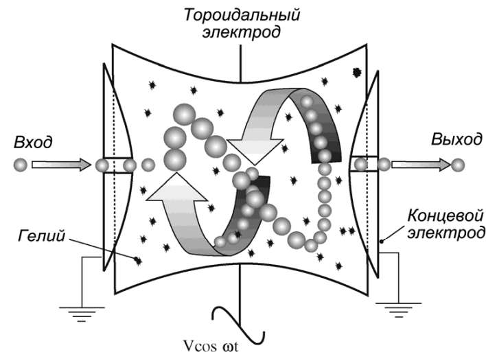
Рисунок 74 – Схема ионной ловушки
