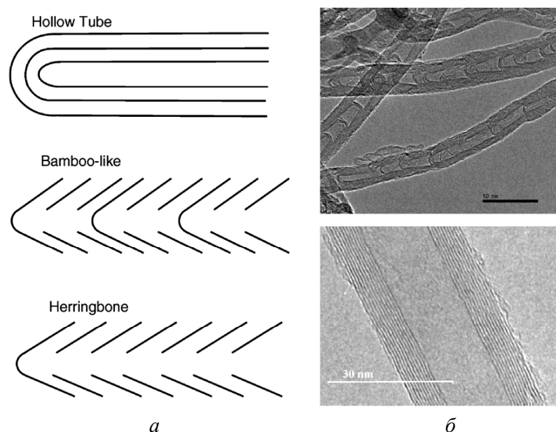
Рисунок 96 – Многостенные углеродные нанотрубки: а – схемы строения нанотрубок; б – электронные микрофотографии бамбукообразных (вверху) и полых (внизу) нанотрубок
