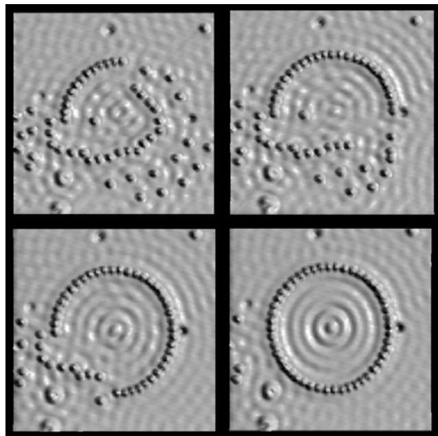
Рисунок 58 – Поэтапное создание кольцевого "коралла" из атомов железа используя атомно-силовой микроскоп ( http://www.almaden.ibm.com/vis/stm/corral.html )
