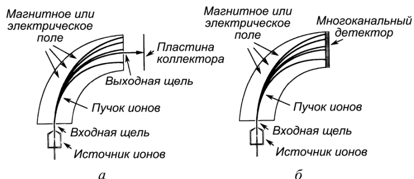
Рисунок 70 – Схема секторных масс-спектрометров: а – с одноканальным детектором, б – с многоканальным детектором
