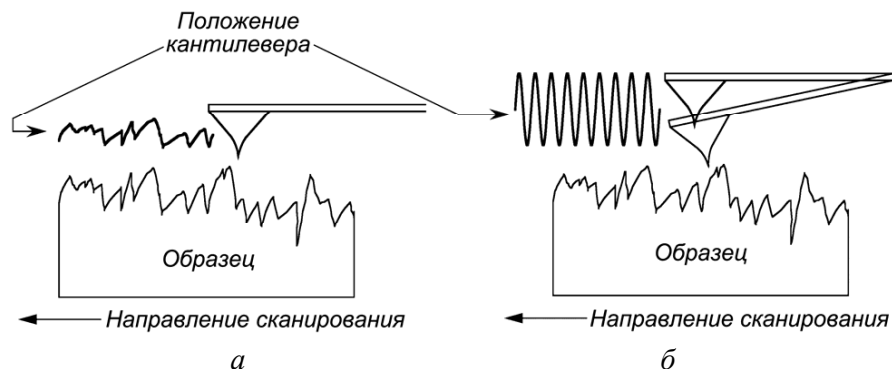
Рисунок 56 – Два режима сканирования: а – контактный; б – динамический
