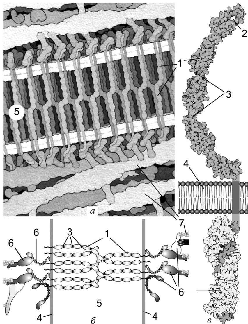
Рисунок 194 – Межклеточное соединение с помощью белков кадхеринов
