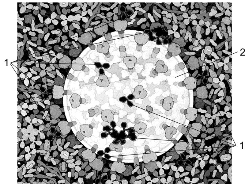
Рисунок 25 – Связывание антител белками липопротеидной оболочки вируса: 1 – антитела; 2 – вирион ВИЧ
