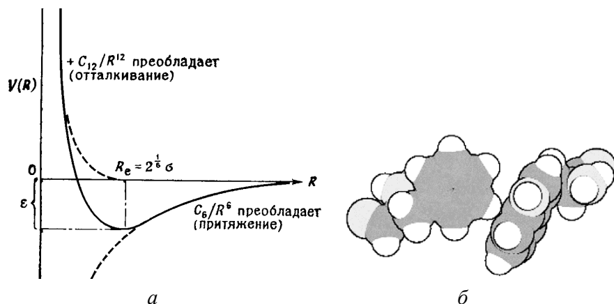
Рисунок 111 – Ван-дер-ваальсовое взаимодействие: a – потенциал Ленарда-Джонса; б – ван-дер-ваальсовое представление молекулярного комплекса
