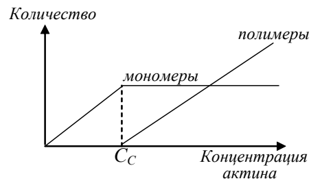
Рисунок 179 – Зависимость количества мономеров и полимеров от концентрации актина
