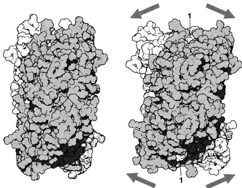
Рисунок 174 – Аллостерическое изменение фермента фруктозо-1,6-бифосфатаза в результате связывания молекул-эффекторов. 1 – эффектор. Стрелками показаны направления смещения субъединиц фермента
