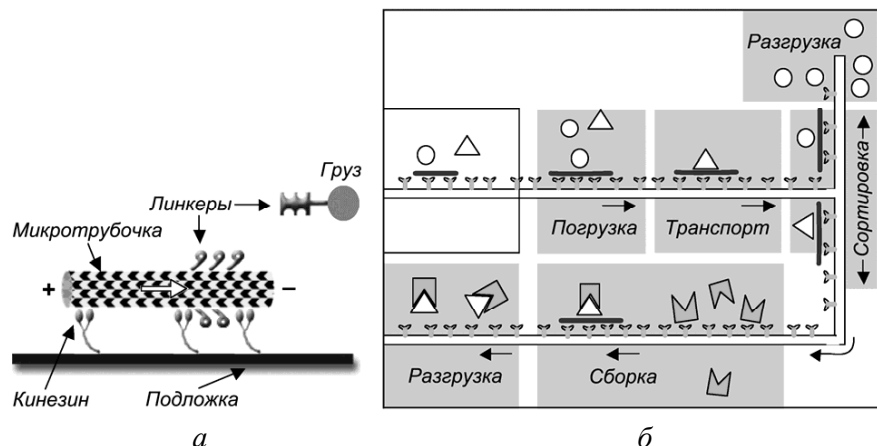
Рисунок 257 – Молекулярный шаттл: а – схема транспортного шаттла; б – схема нанотранспорта молекулярными шаттлами
