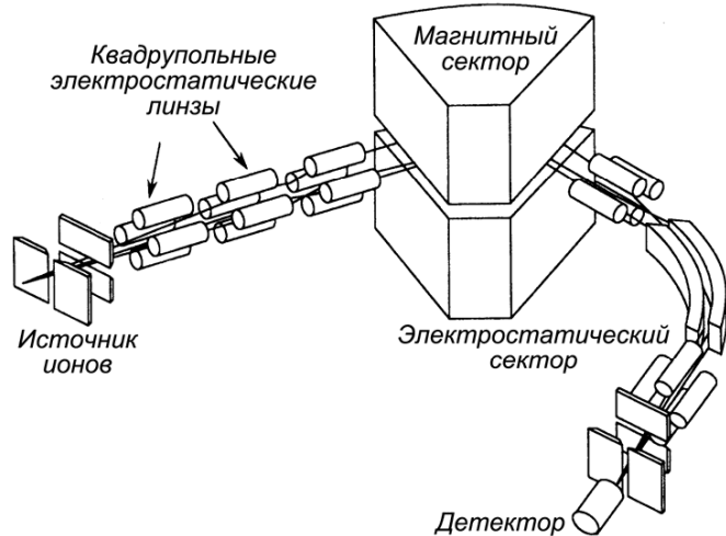
Рисунок 71 – Схема двухфокусного масс-спектрометра
