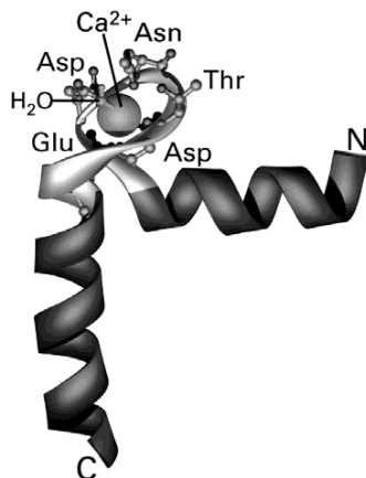
Рисунок 12 – Схема одного из четырёх кальций-связывающих мотивов спираль-петля-спираль кальмодулина
