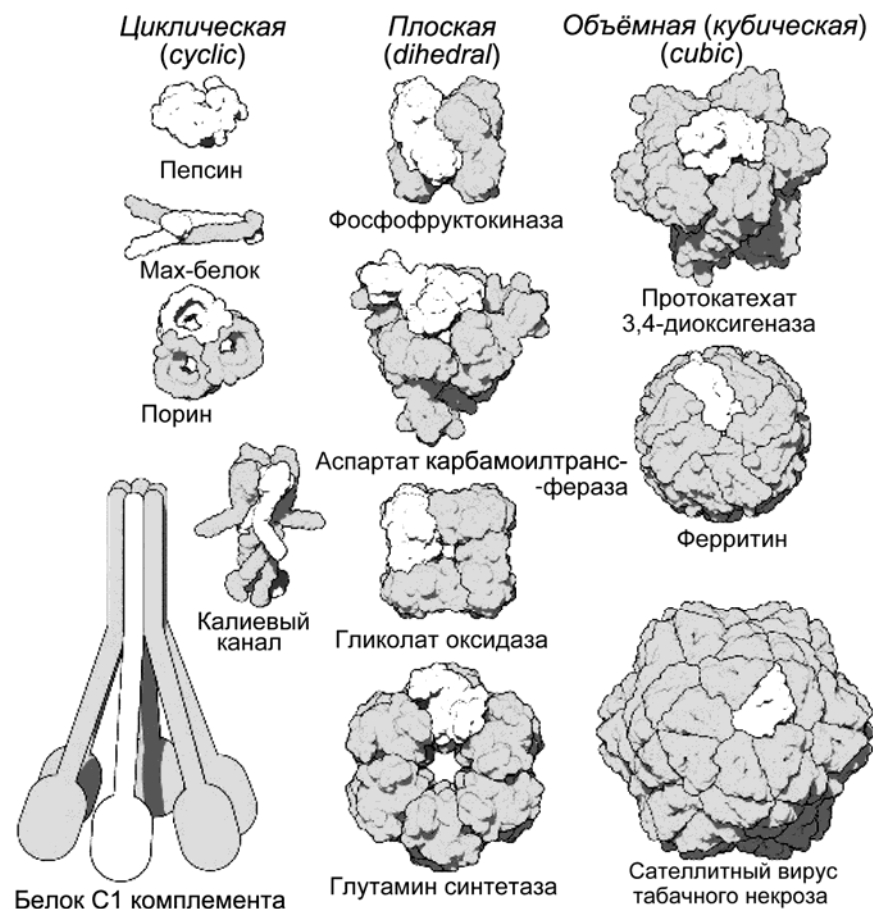
Рисунок 130 – Симметрия биомолекул
