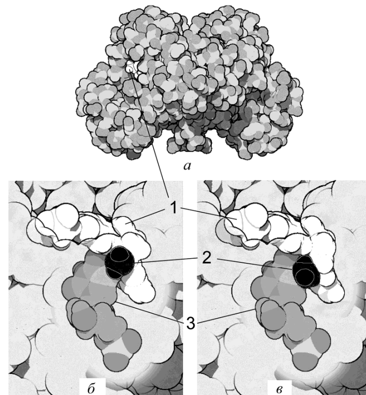
Рисунок 18 – Фермент тимидилат синтаза: а – схема молекулы, кофактор (белый) расположен в левом верхнем кармане фермента; б – исходное расположение молекул перед каталитическим актом, метильная группа связана с кофактором; в – расположение молекул после катализа, метильная группа присоединена к нуклеотиду; 1 – кофактор; 2 – метильная группа; 3 – тимидин
