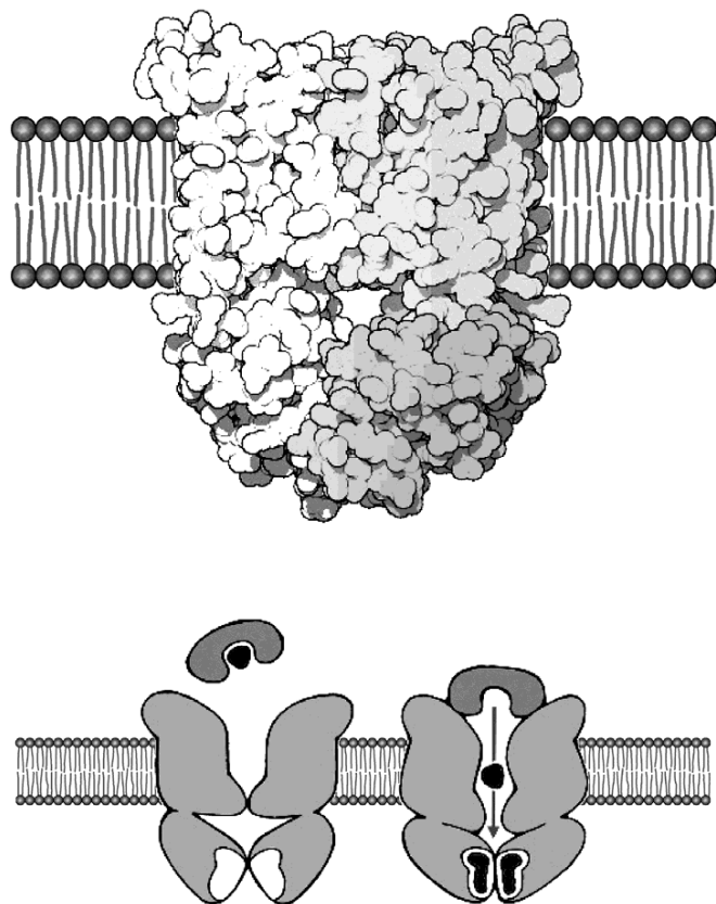
Рисунок 210 – Схема работа бактериального BtuCD-транспортёра
