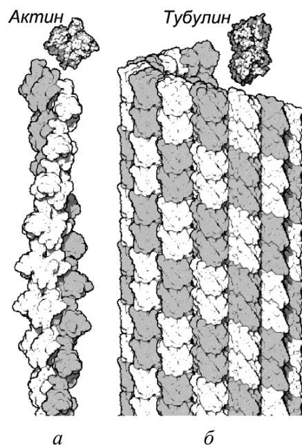
Рисунок 134 – Наиболее распространенные спиральные бионаноструктуры: а – актиновая нить, б – микротрубочка
