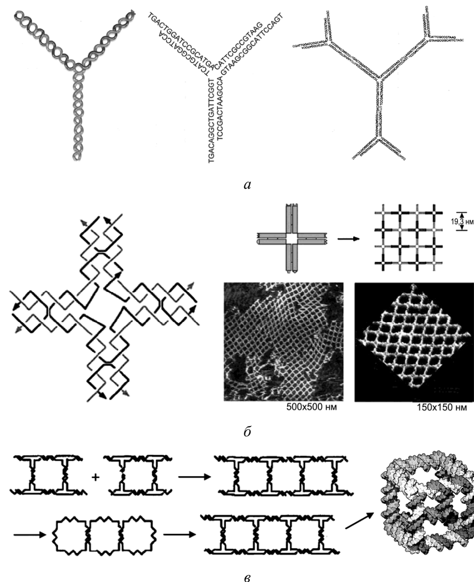
Рисунок 251 – Формирование ДНК-структур: а – схема элемента Y-ДНК и сборки дендримера из четырёх Y-ДНК; б – схема 4×4 ДНК-блока и сборки прямоугольных решёток из 4×4-блоков; в – ассемблирование ДНК-нанокуба
