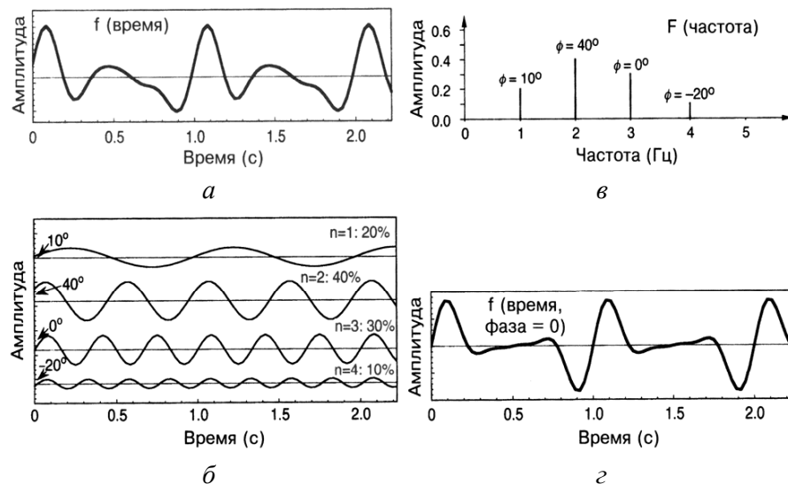
Рисунок 38 – Пример одномерного преобразования Фурье
