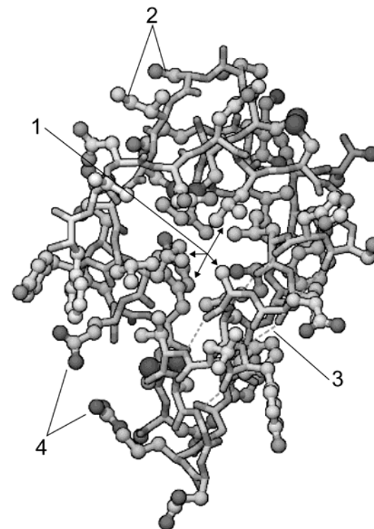
Рисунок 105 – Физические взаимодействия в молекуле инсулина: 1 – гидрофобные аминокислоты (гидрофобный эффект); 2 – ковалентные связи; 3 – водородные связи; 4 – заряженные аминокислоты (электростатические взаимодействия)
