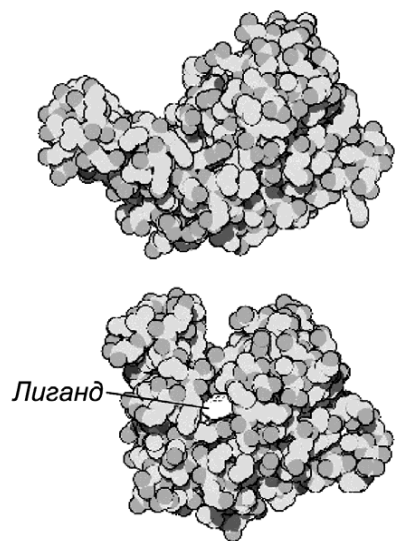
Рисунок 151 – Индуцированное соответствие на примере аденилат-киназы
