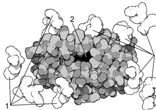
Рисунок 103 – Моделирование молекулярного докинга молекул лекарственного препарата саквинавир ( saquinavir ) к ВИЧ-протеазе: 1 – различные конформации молекул саквинавира; 2 – наиболее "удачная" конформация саквинавира, связанная в активном центре протеазы
