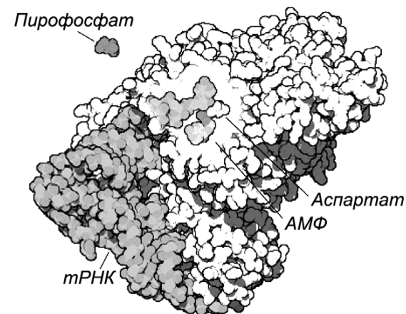
Рисунок 161 – Фермент аспартил-тРНК-синтетаза
