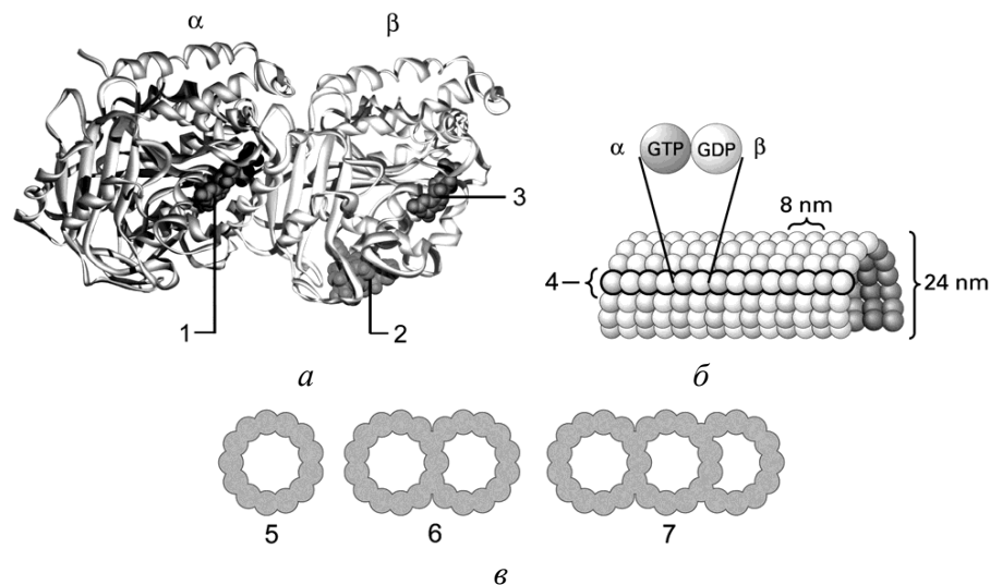
Рисунок 181 – Строение микротрубочек: а – гетеродимер тубулина; б – цилиндрический полимер; в – "упаковка" протофиламентов; 1 – ГТФ (GTP); 2 – молекула таксола ( taxol ); 3 – ГДФ (GDP); 4 – протофиламент; 5–7 – одинарные, двойные и тройные микротрубочки
