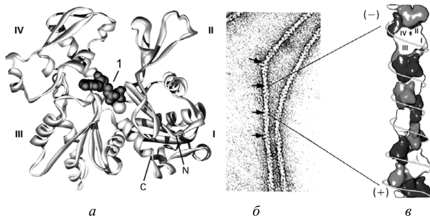
Рисунок 178 – Структура глобулярного и фибриллярного актина: а – модель мономера G-актина; 1 – складка, в которой связывается АТФ, С- и N- концы находятся в субдомене I; б – спираль F-актина в электронном микроскопе; в – модель полимера актина
