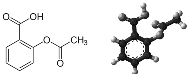
Рисунок 239 – Ацетилсалициловая кислота
