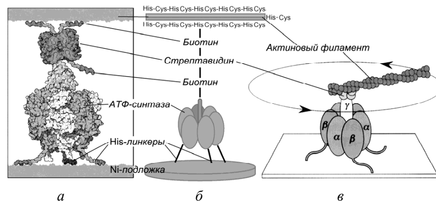
Рисунок 256 – Нановентилятор: a – молекулярная схема; б – схема компоновки узлов; в – схема работы
