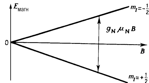
Рисунок 49 – Схема энергетического ЯМР-сдвига уровней в магнитном поле
