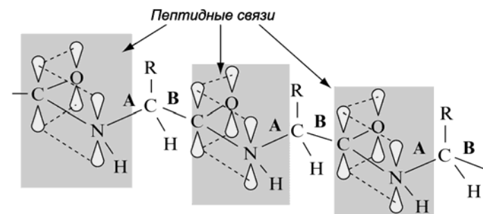
Рисунок 108 – Резонансы в пептидной связи
