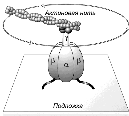
Рисунок 204 – Вращение \gamma -субъединицы АТФ-синтазы
