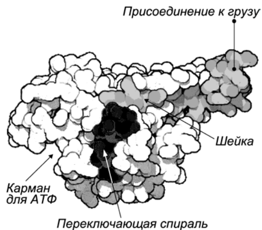
Рисунок 200 – Структура моторной головки кинезина
