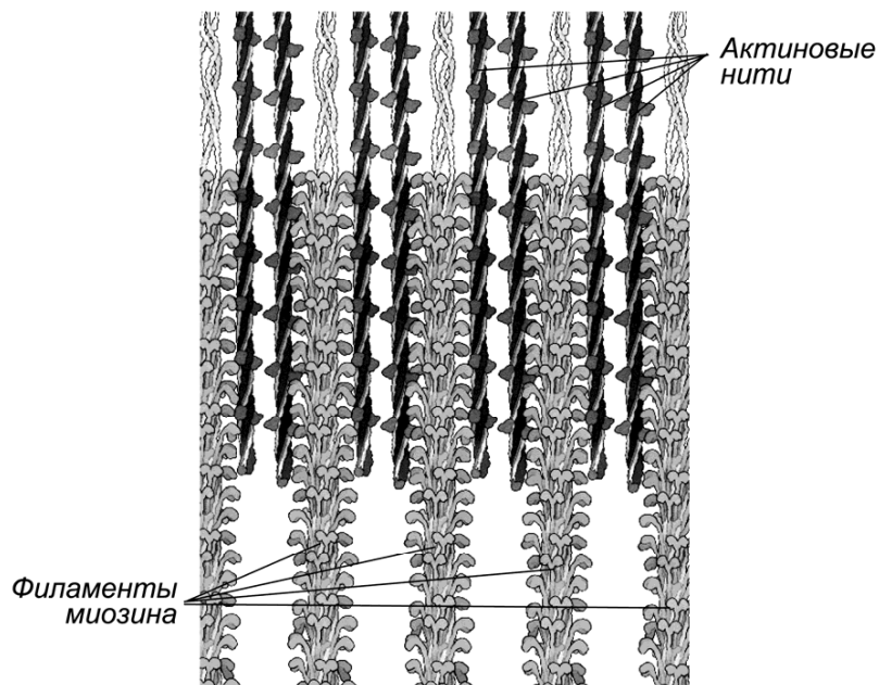
Рисунок 22 – Схема расположения актиновых нитей и миозина в саркомере
