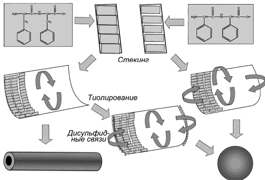
Рисунок 229 – Самосборка нанотрубок и наносфер из дипептидов фенилаланина и фенилглицина
