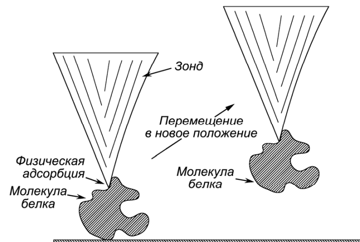
Рисунок 57 – Манипуляции с молекулой белка с помощью атомно-силового микроскопа
