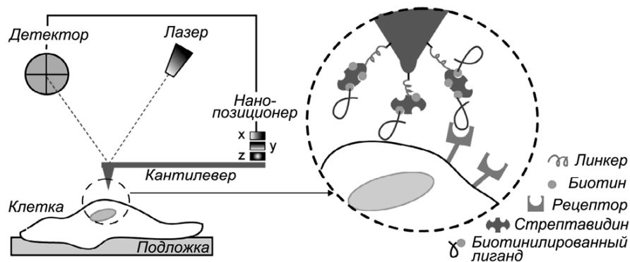
Рисунок 86 – Измерение силы межмолекулярного взаимодействия мембранного рецептора клетки с соответствующим лигандом
