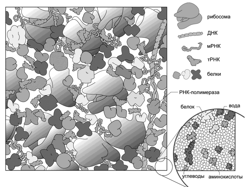
Рисунок 138 – Содержимое бактериальной клетки Escherichia coli
