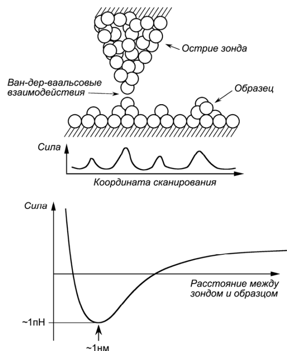
Рисунок 55 – Взаимодействие зонда кантилевера с образцом
