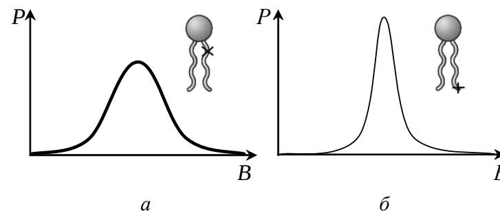
Рисунок 48 – Два способа прикрепления спиновой метки к фосфолипидной молекуле и различие спектров ЭПР для этих двух случаев (схематичное изображение)
