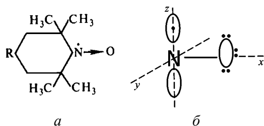
Рисунок 47 – Спиновые зонды: a – формула спинового зонда 2,2,6,6-тетраметилпиперидин-1-оксин (ТЕМПО); b – схема электронного строения парамагнитного фрагмента нитроксильного радикала
