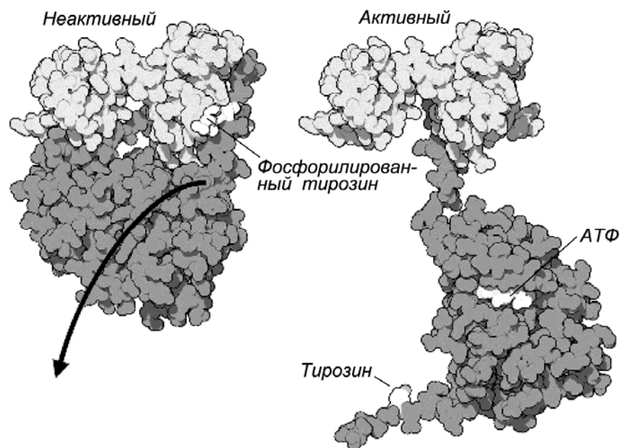
Рисунок 175 – Регулирование активности белка SRC-тирозин-киназа фосфорилированием
