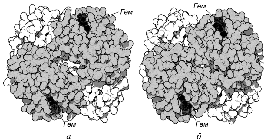
Рисунок 149 – Конформации гемоглобина при связывании молекулы кислорода: а – гемоглобин без кислорода, б – оксигенизированный гемоглобин
