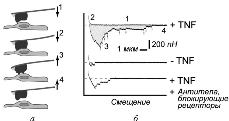
Рисунок 88 – Измерение силы межклеточной адгезии
