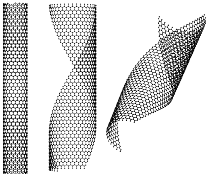
Рисунок 93 – Сворачивание графенового листа в углеродную нанотрубку
