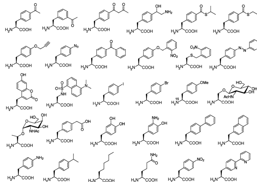
Рисунок 221 – Нестандартные аминокислоты
