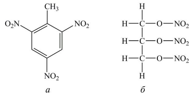
Рисунок 159 – Топливные молекулы: а – 2,4,6-тринитротолуол (ТНТ, тротил), б – нитроглицерин (тринитрат глицерина)
