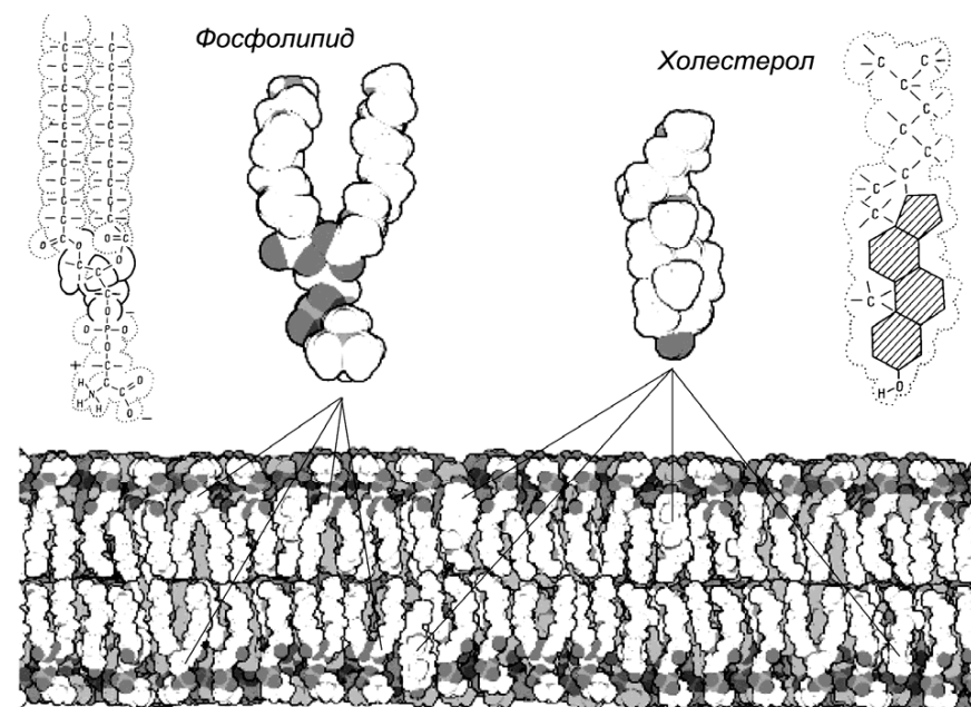
Рисунок 16 – Молекулы фосфолипида (фосфатидилсерин) и холестерина из которых происходит самосборка биомембраны. Темно-серым цветом обозначены полярные участки молекул
