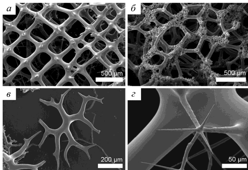
Рисунок 188 – Примеры кремнистых скелетов губок
