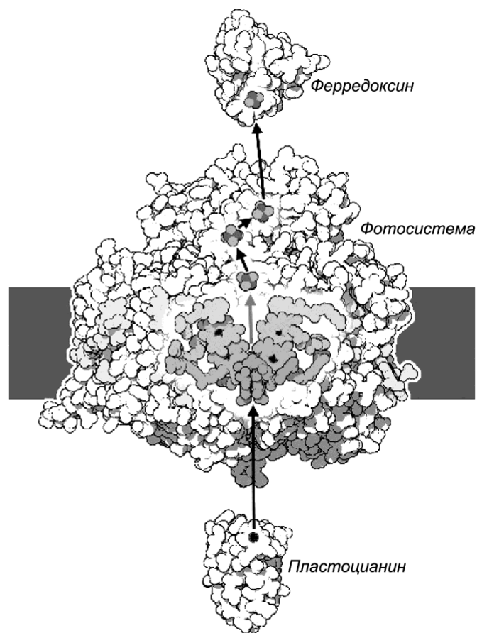
Рисунок 163 – Фотосинтетический реакционный центр цианобактерии
