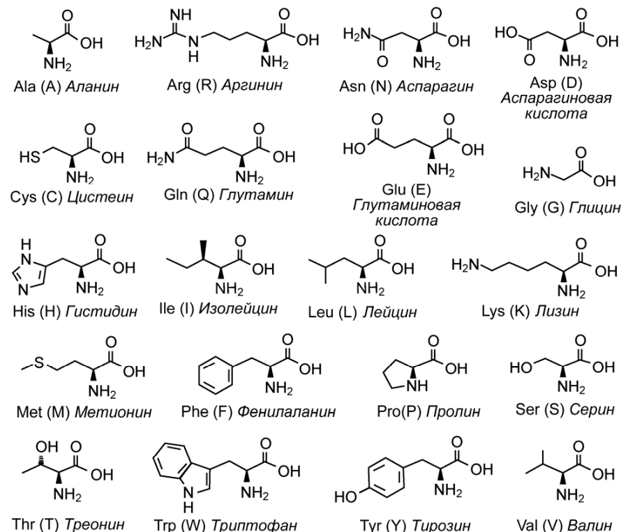
Рисунок 4 – Стандартные аминокислоты
