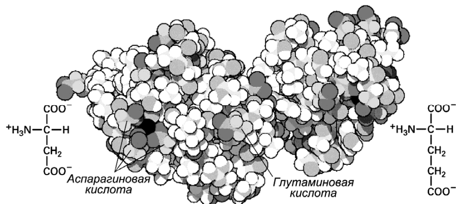
Рисунок 11 – Структурные особенности аспарагиновой и глутаминовой кислот
