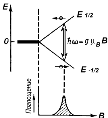
Рисунок 45 – Схема энергетического сдвига уровней в магнитном поле и формирования линии в спектре ЭПР
