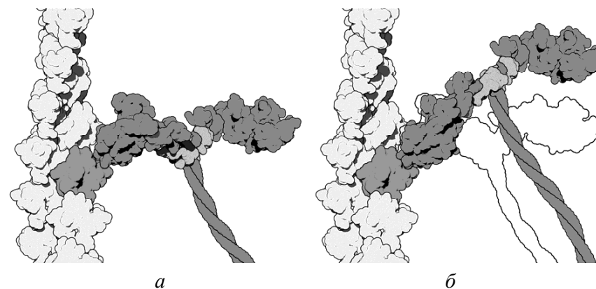
Рисунок 196 – Рабочий ход миозина: а – начало; б – конец рабочего хода
