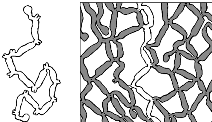
Рисунок 193 – Структура эластина
