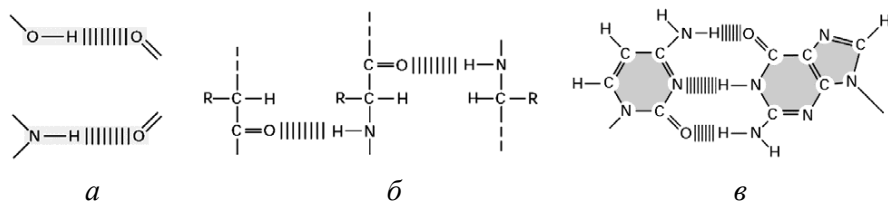
Рисунок 114 – Внутримолекулярные водородные связи в белках и нуклеиновых кислотах: а – сила связи наибольшая при линейном расположении атомов; б – водородные связи между полипептидными цепями белков; в – азотистые основания цитозин и гуанин в ДНК спариваются, образуя водородные мостики
