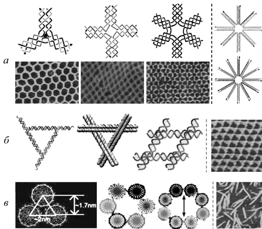
Рисунок 252 – ДНК-сборки: а – 3-, 4- и 6-лучевые ДНК-блоки и сборки из них; б – треугольные и ромбические ДНК-блоки и сборка из них; в – 3-, 6- и 8-ДНК-пучки
