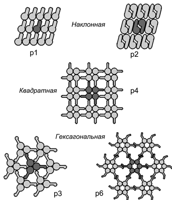
Рисунок 135 – Способы организации S-слоёв
