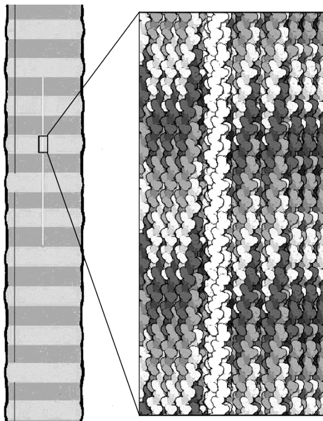
Рисунок 26 – Схема строения коллагенового волокна
