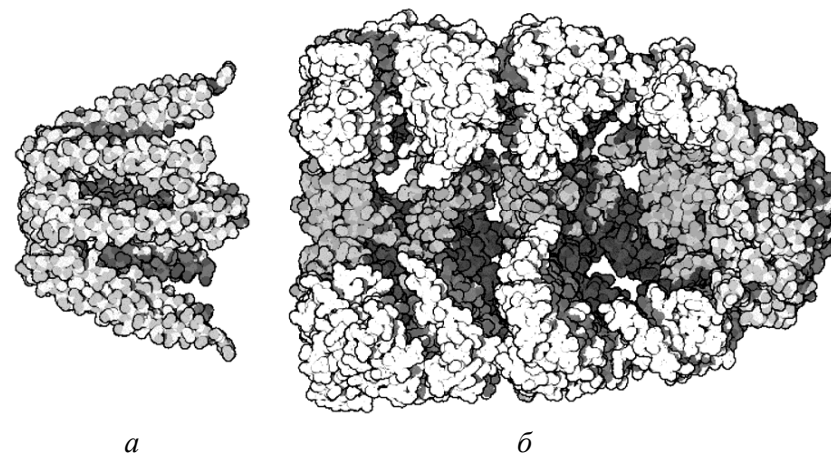
Рисунок 124 – Белки, которые обеспечивают фолдинг: а – перфолдин, б – бактериальный шаперонин GroEL
