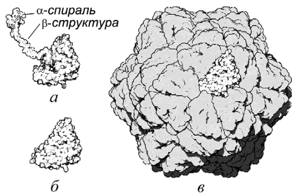
Рисунок 120 – Иерархия белковых структур: а – вторичные структуры, б – третичная структура глобулярного белка, в – четвертичная структура белкового олигомерного вирусного капсида, асSEMBлированного из 60 идентичных субъединиц
