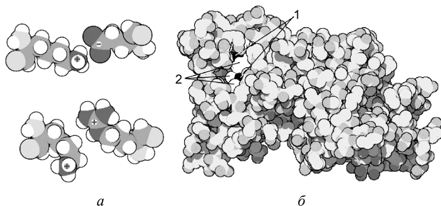
Рисунок 116 – Электростатическое взаимодействие в биомолекулах: а – сверху – лизин и глутаминовая кислота притягиваются, внизу – лизин и аргинин отталкиваются; б – схема фермента супероксид-дисмутаза, обеспечивающего детоксикацию: 1 – ионы меди и цинка в активном центре фермента связывают и химически модифицируют супероксиды (перекиси), 2 – гистидины, которые удерживают ионы металлов в ферменте
