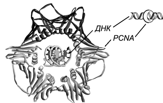
Рисунок 154 – Схема белка PCNA, выполняющего функцию захвата ДНК
