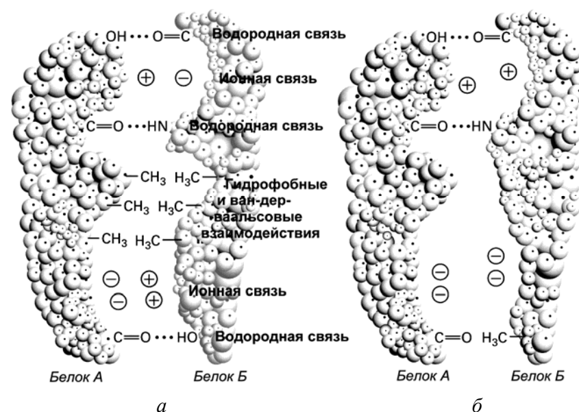
Рисунок 142 – Молекулярное узнавание: а – комплексная комплементарность приводит к образованию прочного комплекса; б – отсутствие комплементарности
