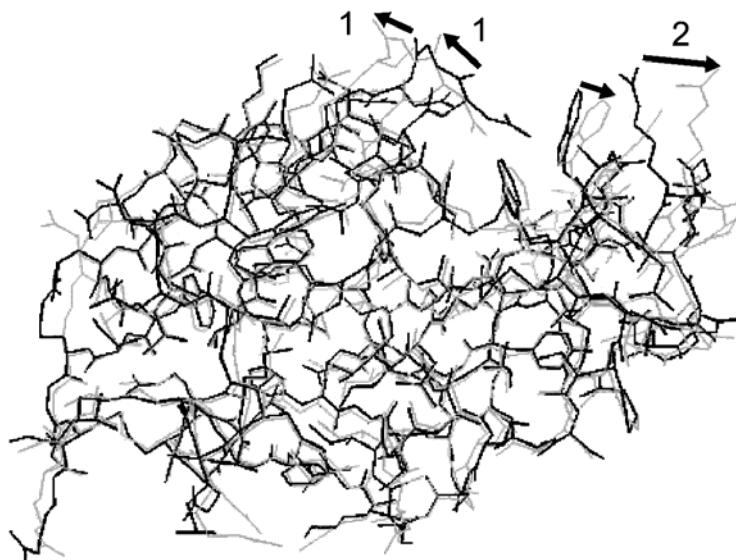
Рисунок 44 – Структура молекулы лизоцима. Стрелками показаны перемещения элементов глобулы: 1 – смещение петли; 2 – движение радикалов аминокислот
