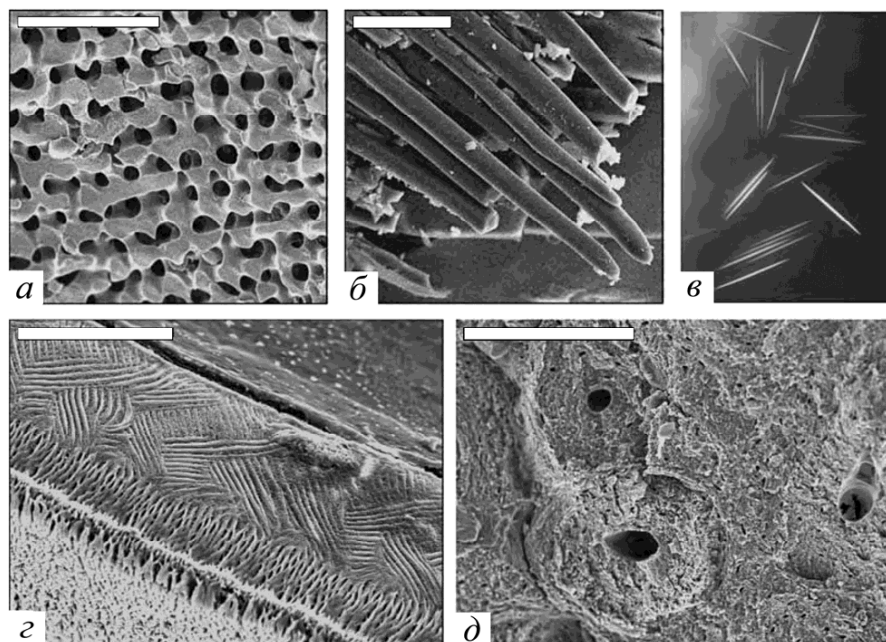
Рисунок 186 – Примеры кальциевой биоминерализации
