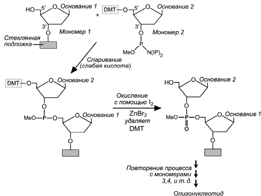
Рисунок 28 – Химический синтез олигонуклеотидов
