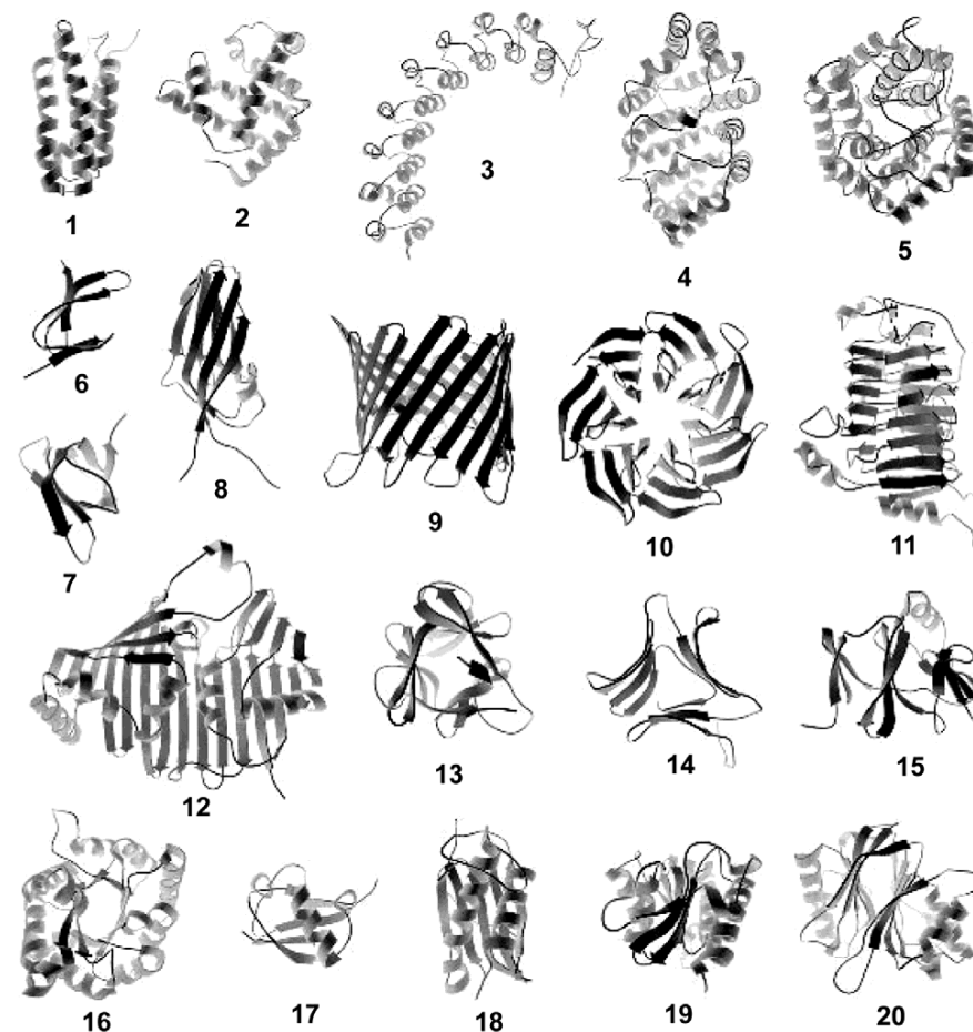
Рисунок 123 – Комбинации \alpha -спиралей, \beta -структур и соединяющих белковых нитей определяют топологию белков: (1–5) – характерные комбинации \alpha -спиралей; (6–15) – характерные комбинации \beta -структур; (16–20) – \alpha/\beta комбинированные комбинации вторичных структур
