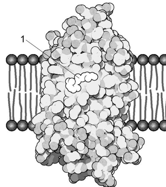
Рисунок 23 – Схема опсина: 1 – молекула ретиналя
