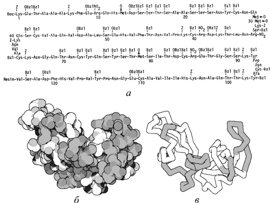
Рисунок 215 – Рибонуклеаза: а – схема первичной структуры с протекторными группами; б – функциональная глобула; в – трассировка полипептидной цепи
