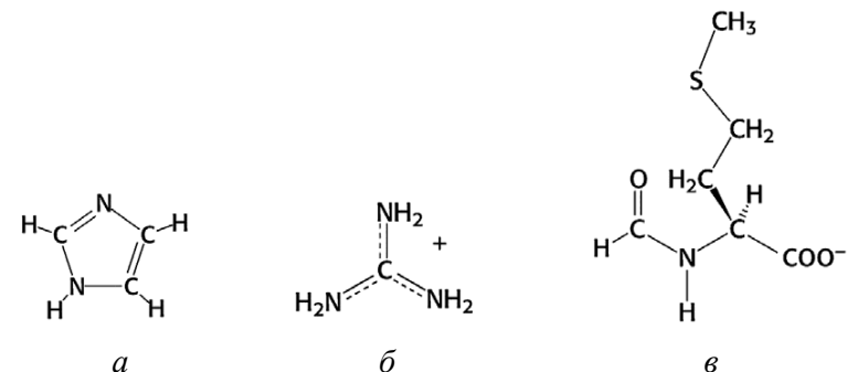
Рисунок 10 – Структурные схемы: а – имидазол; б – гуанидин; в – формилметионин
