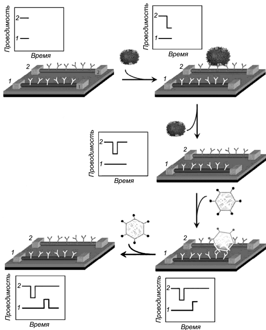
Рисунок 248 – Схема двойного FET-сенсора вирусов
