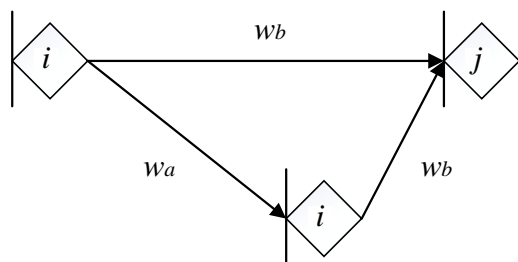
Рис. 5 – Эквивалентный граф
