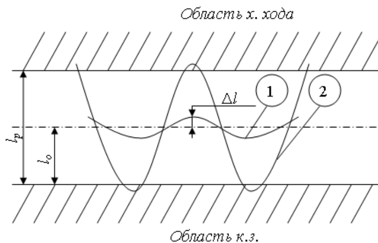
Рис.2. - Режими праці при електроіскрової обробки. 1 - стійкий режим роботи ; 2 - нестійкий режим роботи ; l_p - робочий діапазон переміщення ; l_0 - всталені значення ; \Delta l - величина перерегулювання , \Delta l = (0,1 \dots 0,3) l_p .
