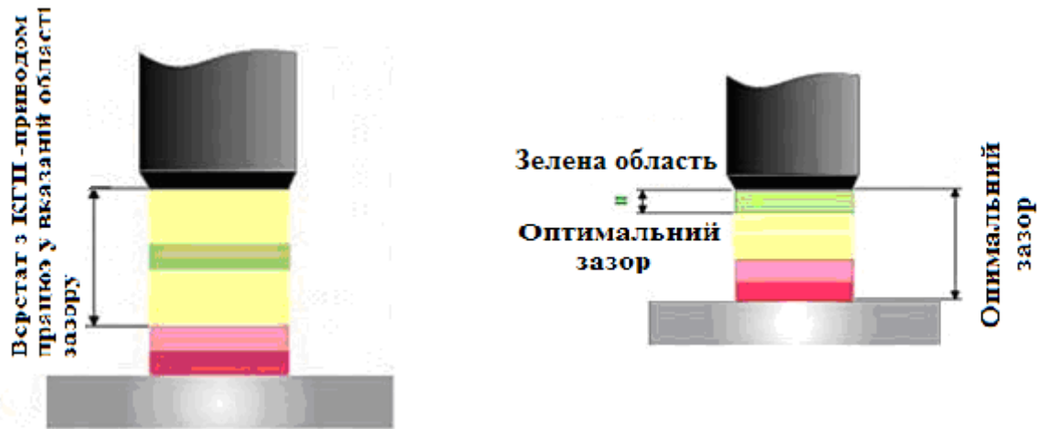
Рис. 1. – Схема порівняння зазорів між електродом та заготовкою в ЕФО-процесі по даним фірми «Sodick».
