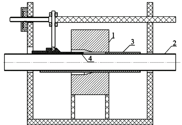
Рисунок 3 – Экспериментальный стенд для измерения распределения индукции магнитного поля на поверхности оболочки: 1 – массивный соленоид, 2 – медная оболочка, 3 – диэлектрическая втулка, 4 – индукционный преобразователь
