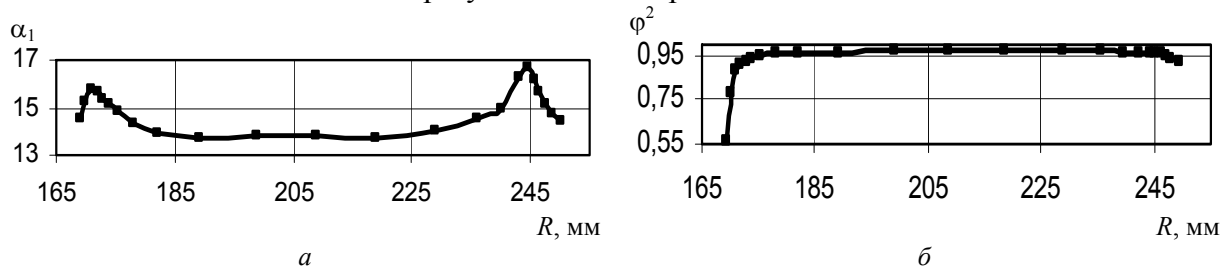
Рис. 2 – Экспериментальные распределения угла потока \alpha_1 а и квадрата коэффициента скорости \varphi^2 б по высоте сечения 1
