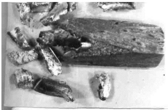
Рис. 5. - Щільно спаковані пакети стружки.
