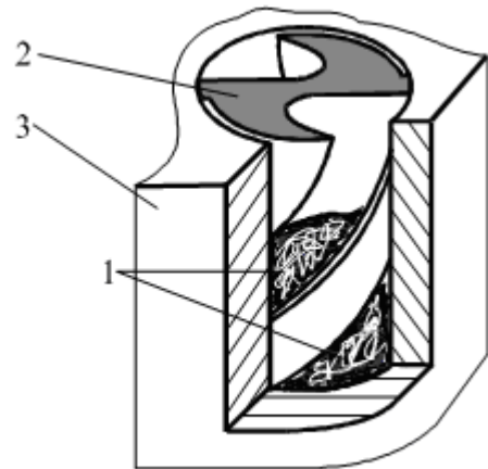
Рис. 6. - Характерні пакети стружки в стружкових канавках спірального свердла \varnothing 11,2 мм при глибині отвору 4-5d. 1 - пакети стружки; 2 - зламане свердло; 3 - деталь з алюмінієвого сплаву.
