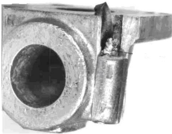
Рис. 6. - Характерні пакети стружки в стружкових канавках спірального свердла \varnothing 11,2 мм при глибині отвору 4-5d. 1 - пакети стружки; 2 - зламане свердло; 3 - деталь з алюмінієвого сплаву.
