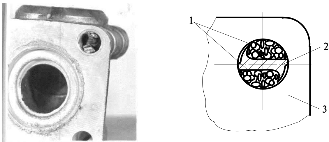
Рис. 1. - Характерна поломка гвинтового свердла \varnothing 11,2 мм в корпусних деталі через пакування стружки в стружкових канавках (матеріал заготовки АК7, інструменту Р6М5Ф3, V = 31,38 мм/хв, S = 0,26 мм/об, охолодження Аквол 10-М 5...7 л/хв. 1 - пакети стружки, 2 - поламане свердло, 3 - деталь з алюмінієвого сплаву.
