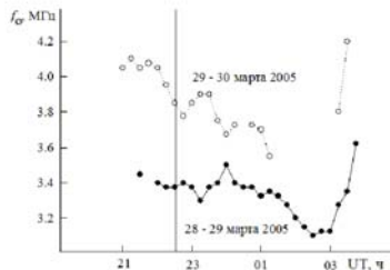
Рис. 1. Зависимость f_oF2 от времени в фоновый период (точки) и в период СР (кружки). На этом и следующих рисунках вертикальной линией показан момент запуска ракеты
