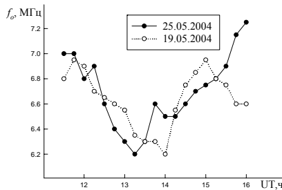
Рис. 3. Зависимость f_0F2 от времени в фоновый период 19 мая 2004 г. (кружки) и в период СР 25 мая 2004 г. (точки)
