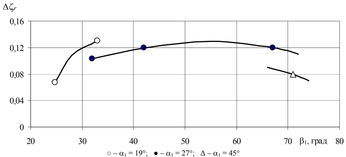
Рис. 3. Влияние радиального зазора на изменение потерь в рабочем колесе \Delta\zeta_r .
