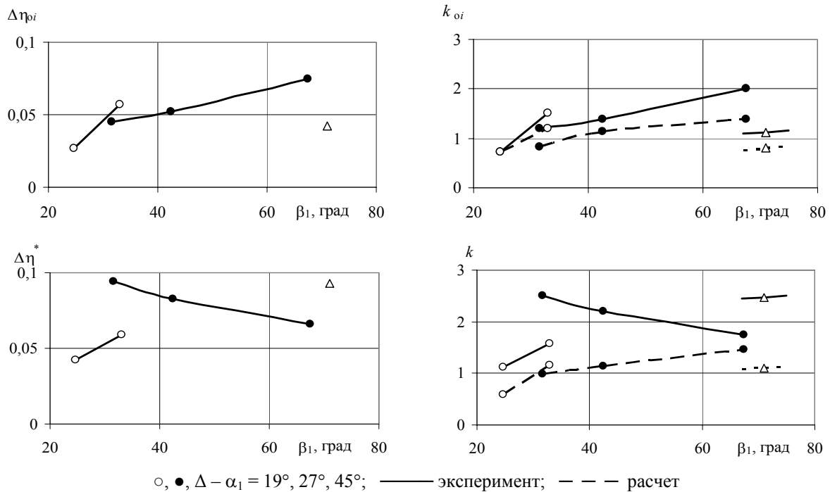
Рис. 2. Влияние изменения радиального зазора от 0,22 мм до 1,0 мм на КПД ступени
