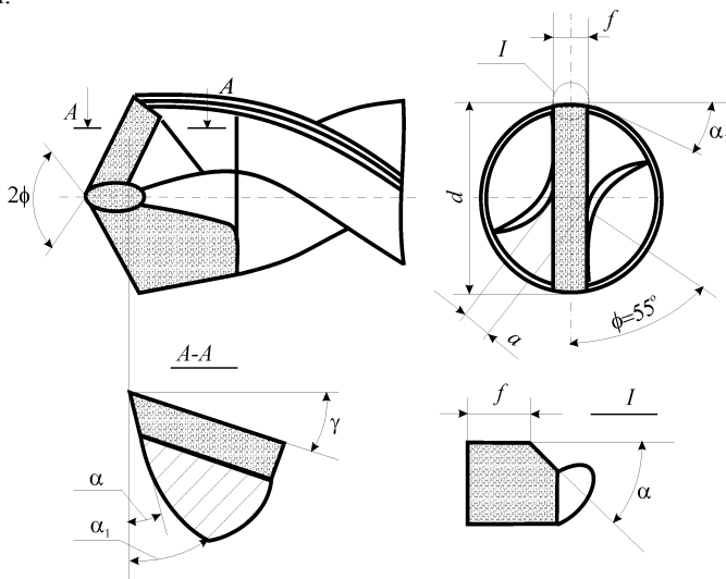
Рисунок 2 – Конструкция сверла из твердого сплава
