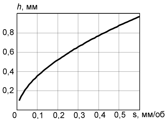
Рисунок 3 – Зависимость глубины начала расслоения от величины подачи
