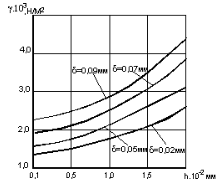
Рис.2. График зависимости коэффициента жёсткости от толщины сдеформированного слоя
