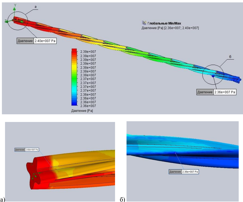
Рис. 1 – Модель поля тиску на поверхні ротора: а – максимальне значення; б – мінімальне значення
