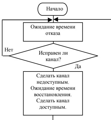
Рис. 2. Логическая схема моделирующего алгоритма отказов
