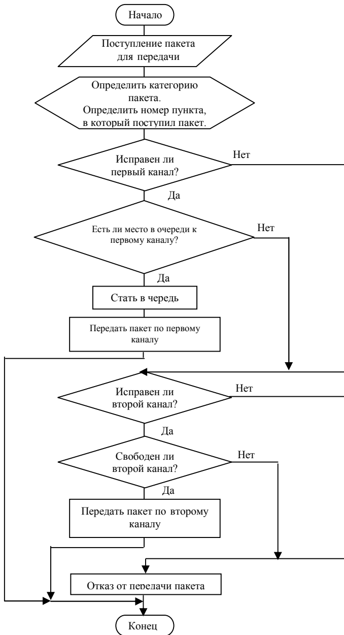
Рис. 3. Логическая схема моделирующего алгоритма системы
