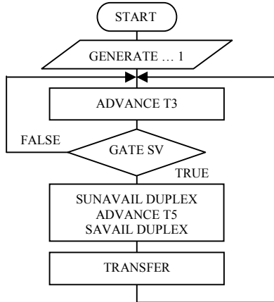
Рис. 5. Схема подпрограммы
