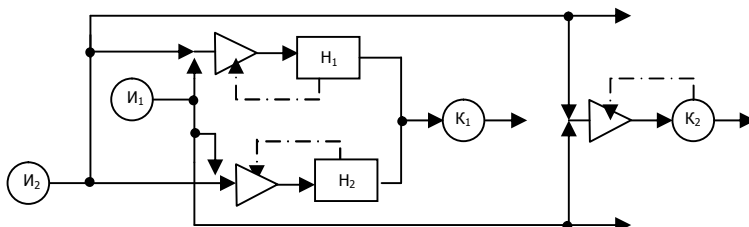
Рис. 1. Структура модели, представленная в виде Q -схемы
