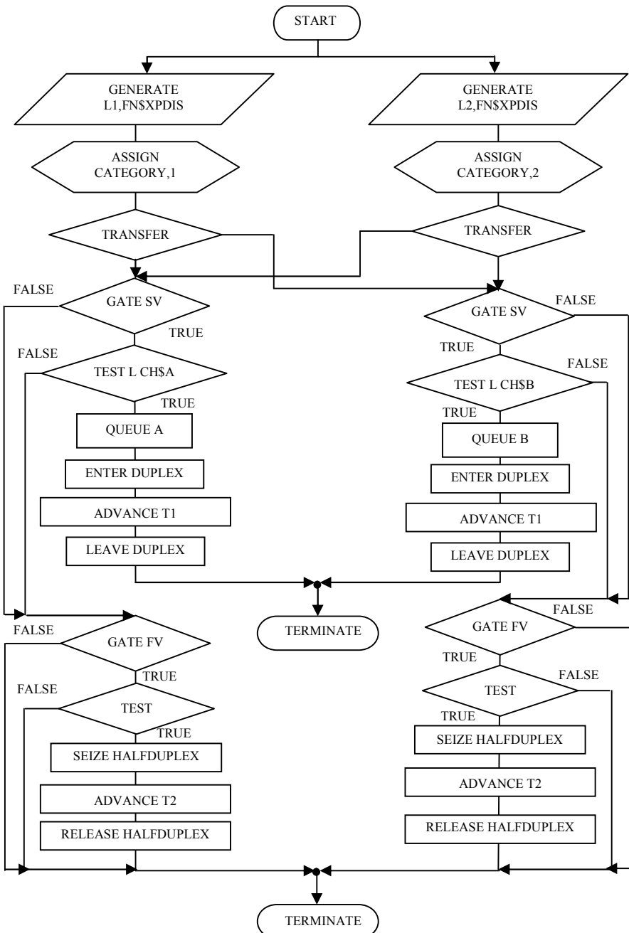
Рис. 4. Схема программы
