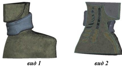
Рисунок 5 – КЭМ с 3-й конструкцией ортеза
