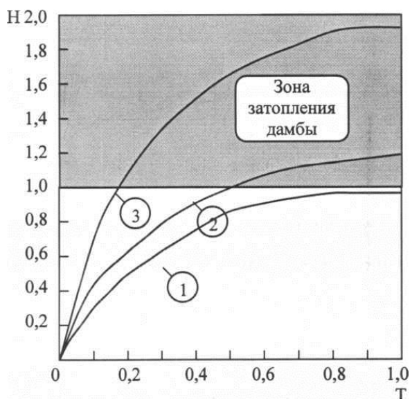
Рис. 2 – Динаміка висоти волни в ВО під совместним впливом смерча F 1.0 и землетрясення: 1 – K_3 = 0 ; 2 – K_3 = 0,3 \cdot 10^3 ; 3 – K_3 = 10^3 .
