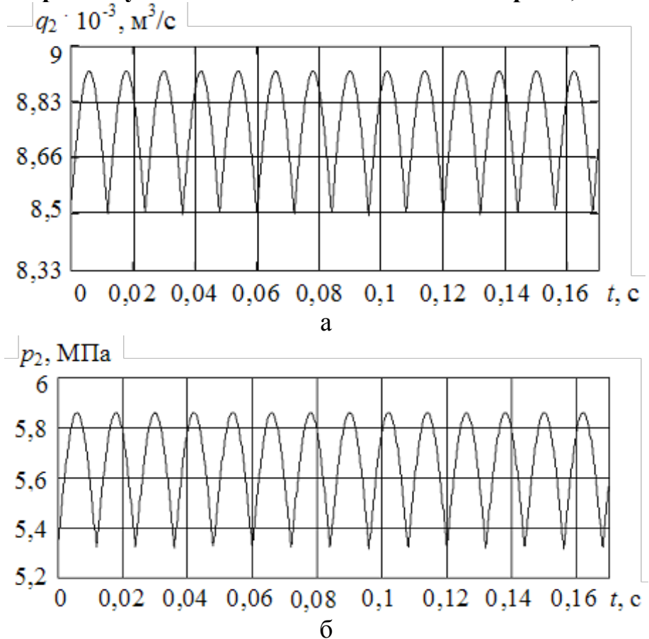
Рис.3. Осцилограми пульсацій у вхідному патрубку 2: а – витрати; б – тиску
