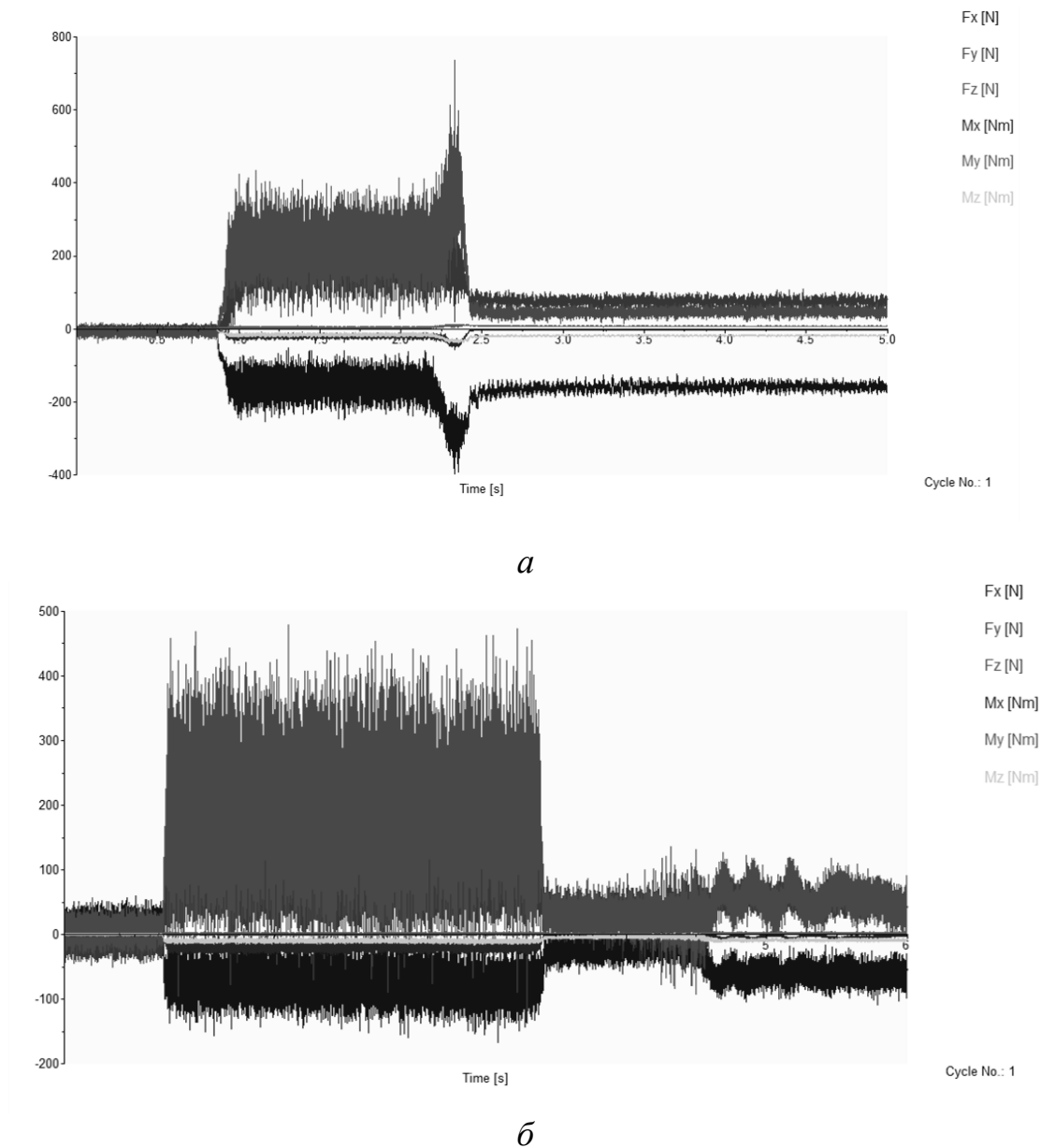
Рис. 3 – Осциллограммы составляющих силы резания ( v = 30 м/мин; s = 0,2 мм/об; t = 0,5 мм): a – КК ВТ6, б – СМК ВТ6
