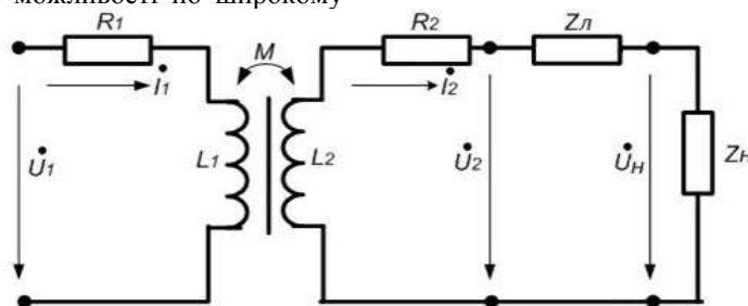
Рис.2 - Схема роботи трансформатора під навантаженням:
