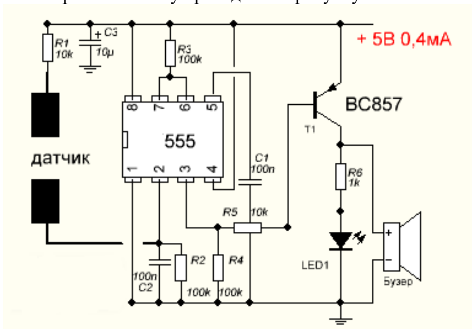
Блок-схема пристрою
