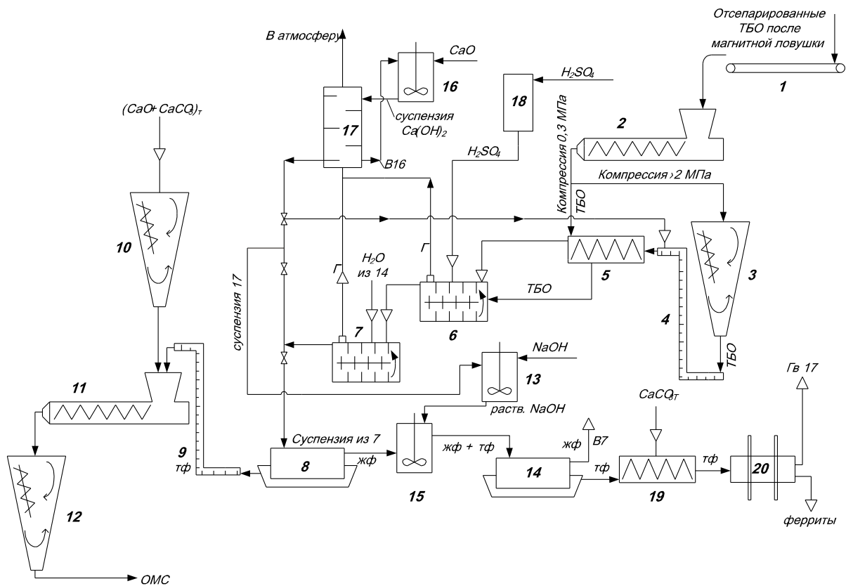
Рис. Принципиальная реакторная схема переработки сепарированных ТБО на ОМС 1 – транспортер-дозатор; 2 – шнековая машина; 3, 10, 12 – бункеры с ворошителями; 4, 9 – редлеры; 5 – шнек-дозатор; 6, 7 – реакторы идеального смешения; 8, 14 – система отстойник-ленточный фильтр-пресс; 11, 19 – шнековый смеситель; 13 – реактор для приготовления раствора NaOH; 15 – реактор для осаждения гидроксидов тяжелых металлов; 16 – емкость для приготовления суспензии \text{Ca}(\text{OH})_2 ; 17 – скруббер для очистки газов; 18 – емкость для \text{H}_2\text{SO}_4 ; 20 – вращающаяся печь
