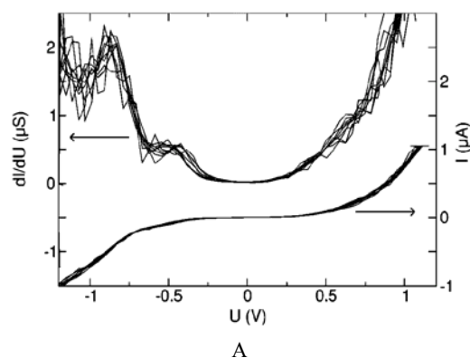
Рис. 12 – Графік зміни провідності в процесі розриву золотого дроту [19]: а – отримані вольтамперні характеристики осадженої органічної молекули; б – формула органічної молекули, що сідає на золоті наноконтакти
