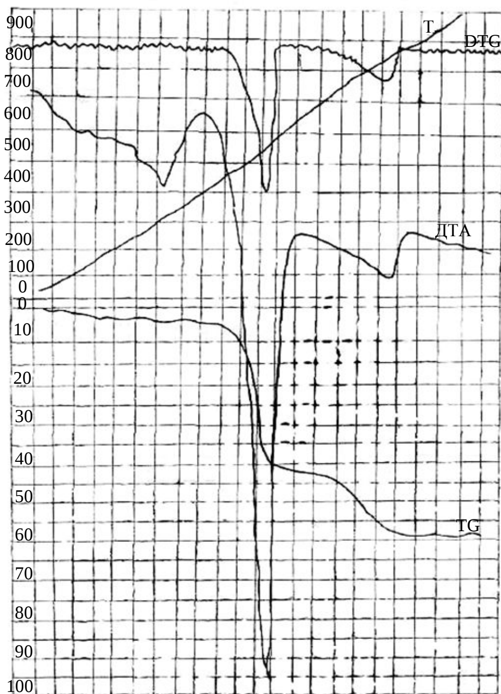
Рис. 1 – Дериватограмма гидроксида кальция, полученного гашением извести избыточным количеством воды до известкового молока.
