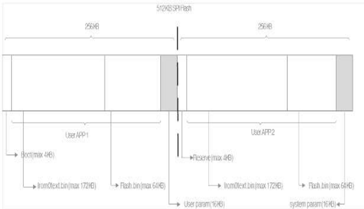
Рис. 2 – Поділ SPI FLASH пам'яті.
