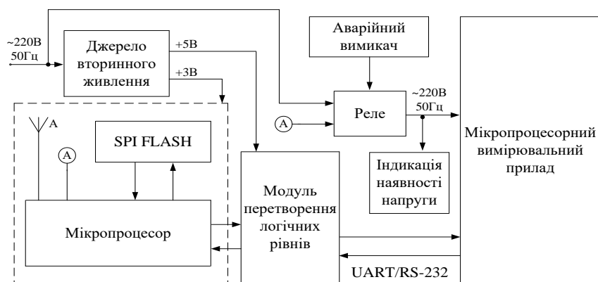
Рис. 1 – Структурна схема системи.
