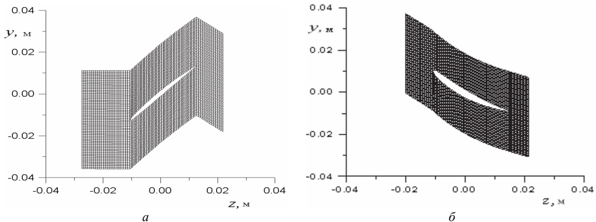
Рис. 4 – Разностная сетка: a – в канале ротора (P1); б – в канале статора (C1)
