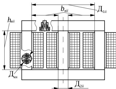
Рис. 2 – Схема поздовжнього перерізу електромагнітної системи реактора з конфігураціями поперечних перерізів стрижня з круговим утворюючим контуром і ярма з плоскою внутрішньою поверхнею
