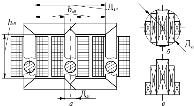
Рис. 1 – Схеми поздовжнього перерізу а – електромагнітної системи трансформатора і конфігурацій поперечних перерізів стрижня та ярма з круговими утворюючими контурами – б і ярма з плоскою внутрішньою поверхнею – в
