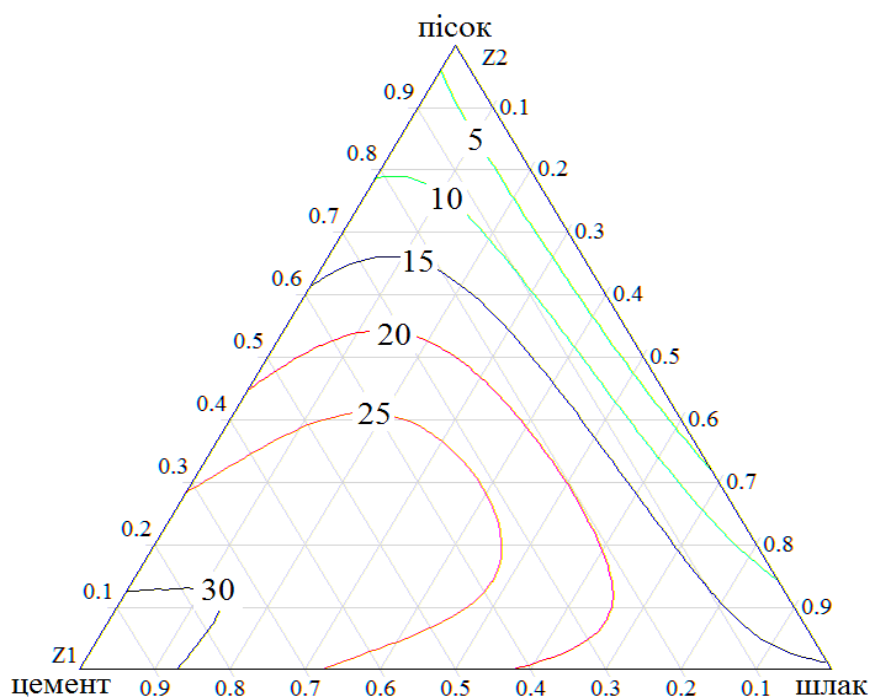
Рис. 3 – Симплекс – діаграма «склад композиції – міцність» та проекції ліній рівного рівня для зразків, що тверднули у воді
