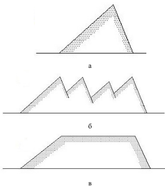
Рис. 3 – виды отвалов: а – конические; б – хребтовые; в – плоские
