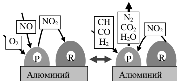
Рис. 3. Схема работы нейтрализатора накопительного типа:
