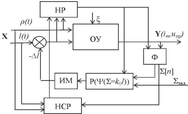
Блок-схема системы управления с НСР
