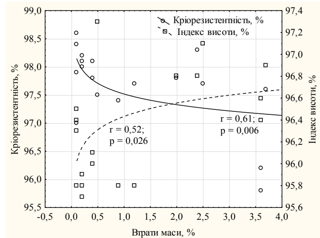
Рис. 3 – Кореляційна залежність кріорезистентності заморожених ягід суниці сорту Дукат та індексу висоти від втрат маси
