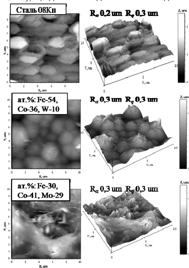
Рис. 1. 2D і 3D-карти поверхні підкладки та покриттів. Площа сканування 10 μm × 10 μm.
