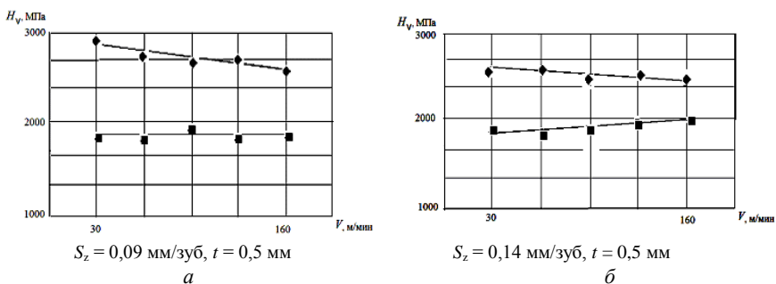
◆ субмикроструктурное состояние; ■ крупнокристаллическое состояние Рисунок 3 – Зависимость микротвердости ВТ1-0 от параметров процесса резания
