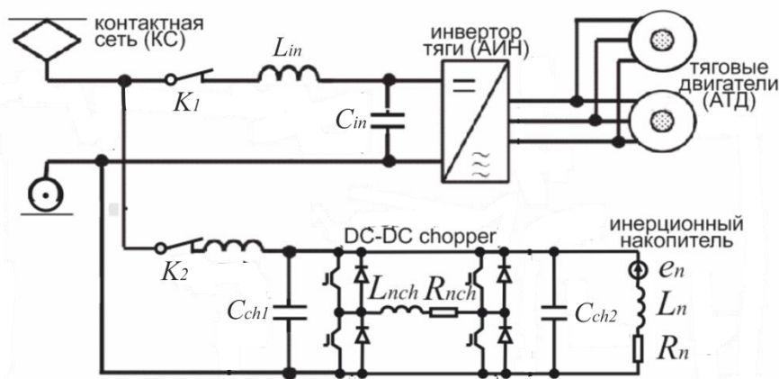
Рис. 2 – Структурная схема тягового агрегата: K_1, K_2 – ключи; L_{in}, L_{ch}, C_{in}, C_{ch1}, C_{ch2} – индуктивности и емкости сетевых фильтров; L_{nch}, R_{nch} – индуктивность и активное сопротивление DC-DC chopper; e_n, L_n, R_n – ЭДС, индуктивность и активное сопротивление накопителя
