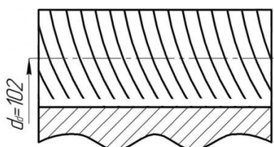
Рисунок 6 – Пятно контакта на зубе парного зубчатого колеса
