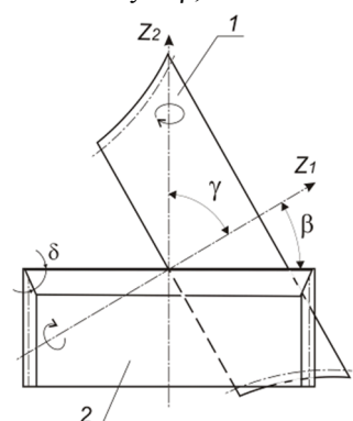
Рисунок 2 – Схема изготовления квазиглобoidного колеса
