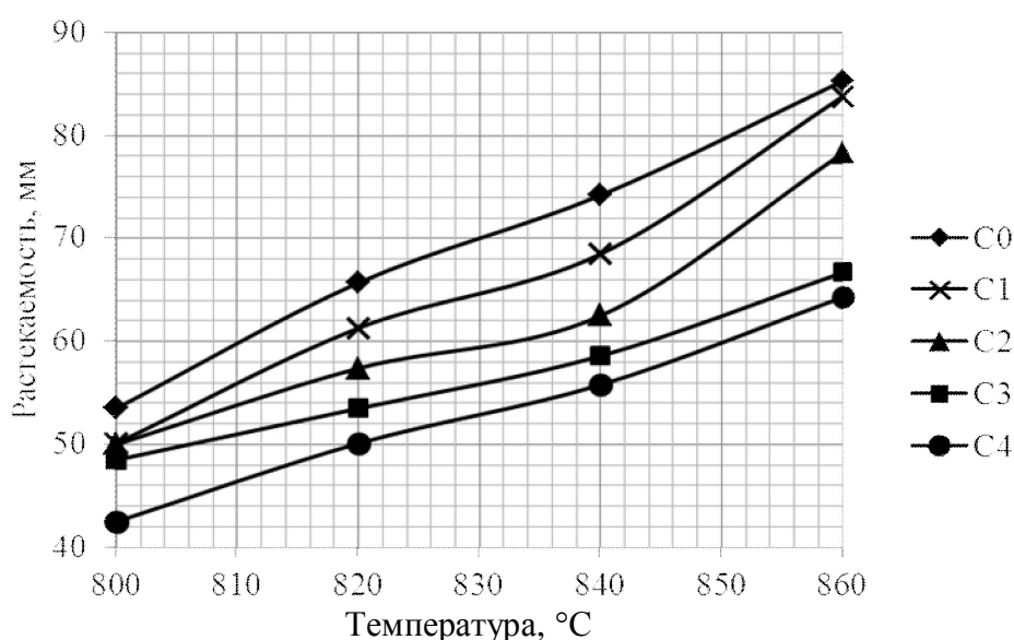
Рис. 2. Растекаемость смесей с различным содержанием песка
