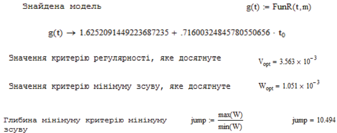
Рис. 4. Вікно програми Mathcad 2000 Professional з результатами пошуку найкращої моделі виду Y = f(X_2)
