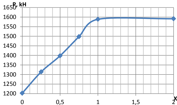
Рис. 2 – Графики зависимости номинального усилия процесса от параметра X при V_2/V_1=1
