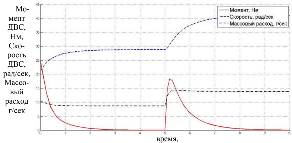
Рис. 1. Результаты моделирования работы ДВС
