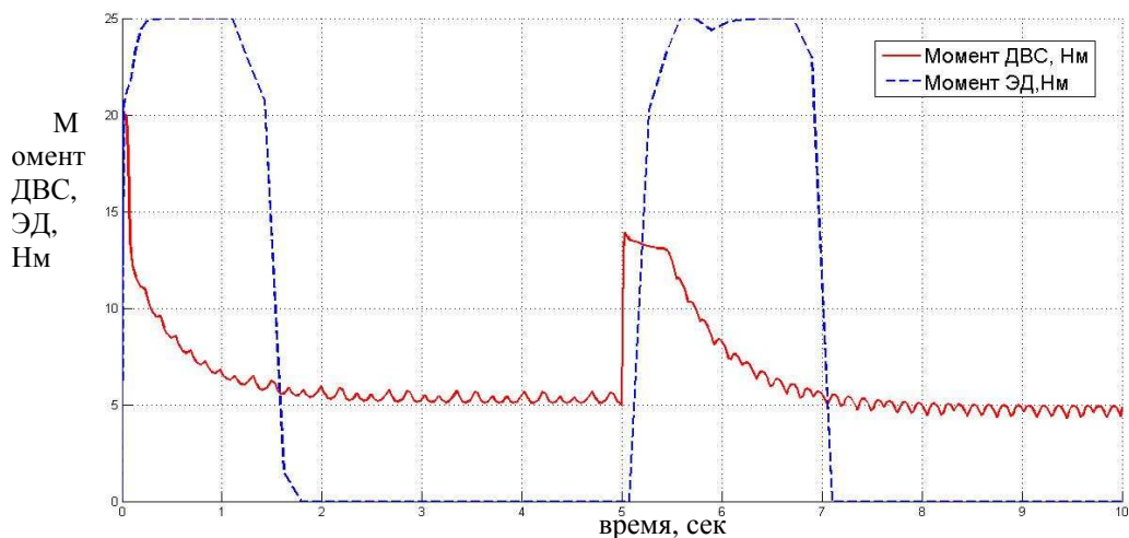
Рис. 2. Совместная работа ДВС и ЭД
