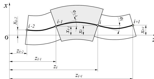
Рисунок 1 – Схема дискретизации вала конечными элементами
