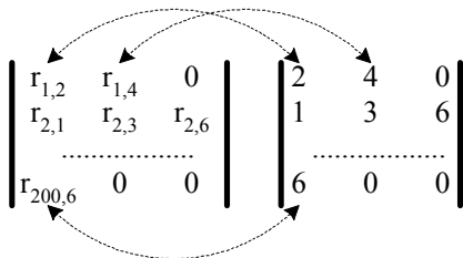
Рисунок 2 – Схема индексации элементов сжатого массива
