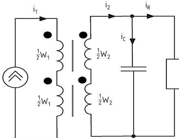
Рис. 1. Трансформаторная схема феррозондового датчика
