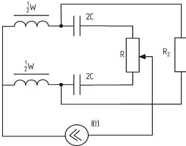
Рис. 2. Мостовая схема феррозондового датчика
