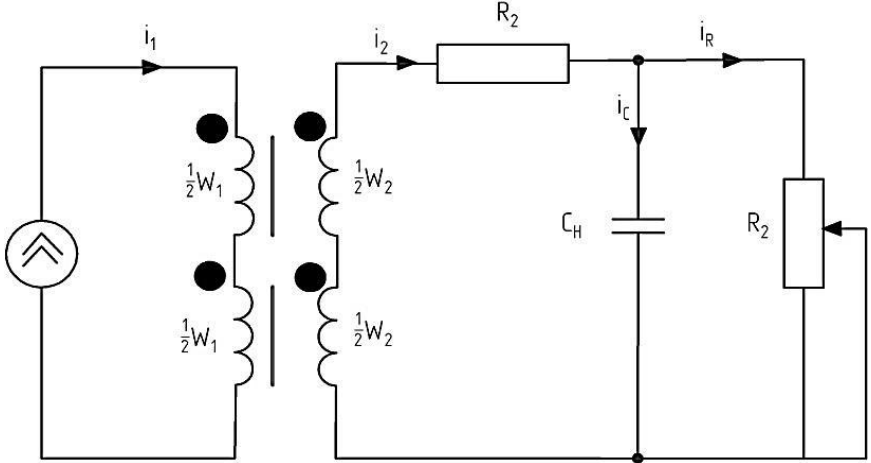
Рис. 3. Обобщенная электрическая схема электромагнитного модулятора
