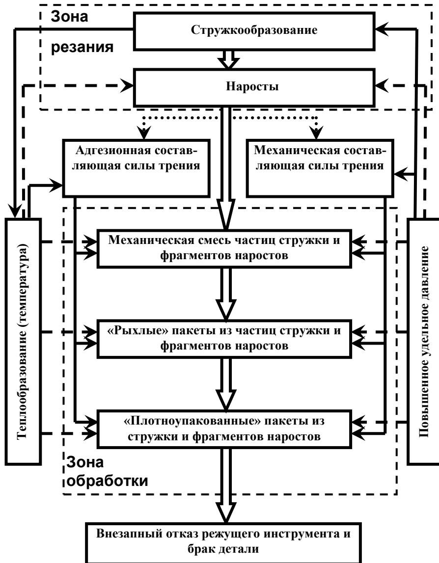
Рис. – Физическая модель процесса образования, транспортирования и пакетирования стружки в стружечных канавках сверл при глубоком сверлении.
