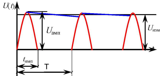
Рис. 7. Принцип работы амплитудного выпрямителя
