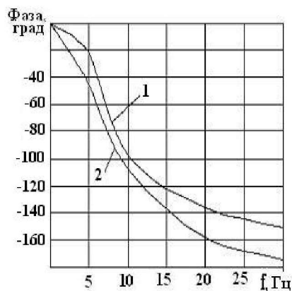
Рис. 7. Фазовая частотная характеристика
