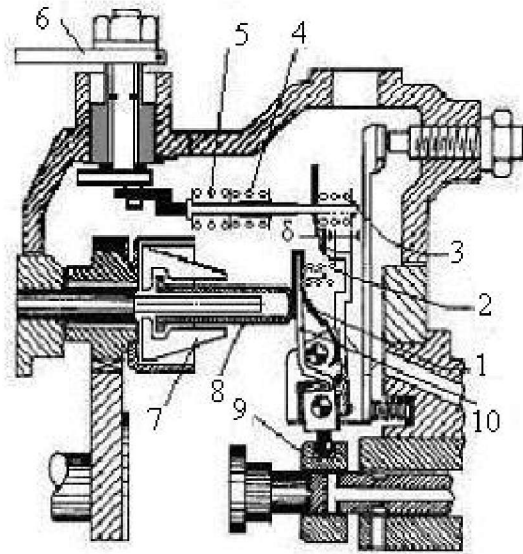
Рис. 1. Схема регулятора
