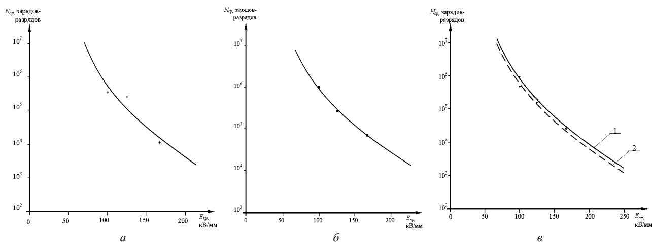
Рисунок 1 – Зависимости длительной электрической прочности от величины рабочей напряженности электрического поля: а – в бумажном диэлектрике, пропитанном касторовым маслом; б – в бумажно-пленочном диэлектрике, пропитанном касторовым маслом; в – в пленочном диэлектрике, пропитанном полиметилсилоксановой жидкостью ПМС-20: 1 – с шоопированными торцами; 2 – со вставными токовыводами.
