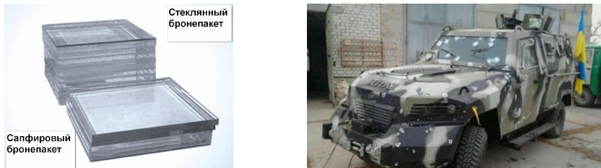
Рис. 1. Сравнение обычного бронестеклянного пакета и прозрачной брони на основе сапфира с одинаковым классом защиты (слева), расстрелянный бронемобиль "Когуар" с окнами из бронестекла (справа)
