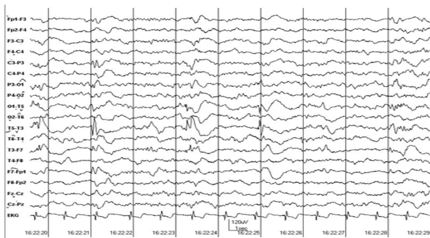
Рис. 1 – Пример ЭЭГ
