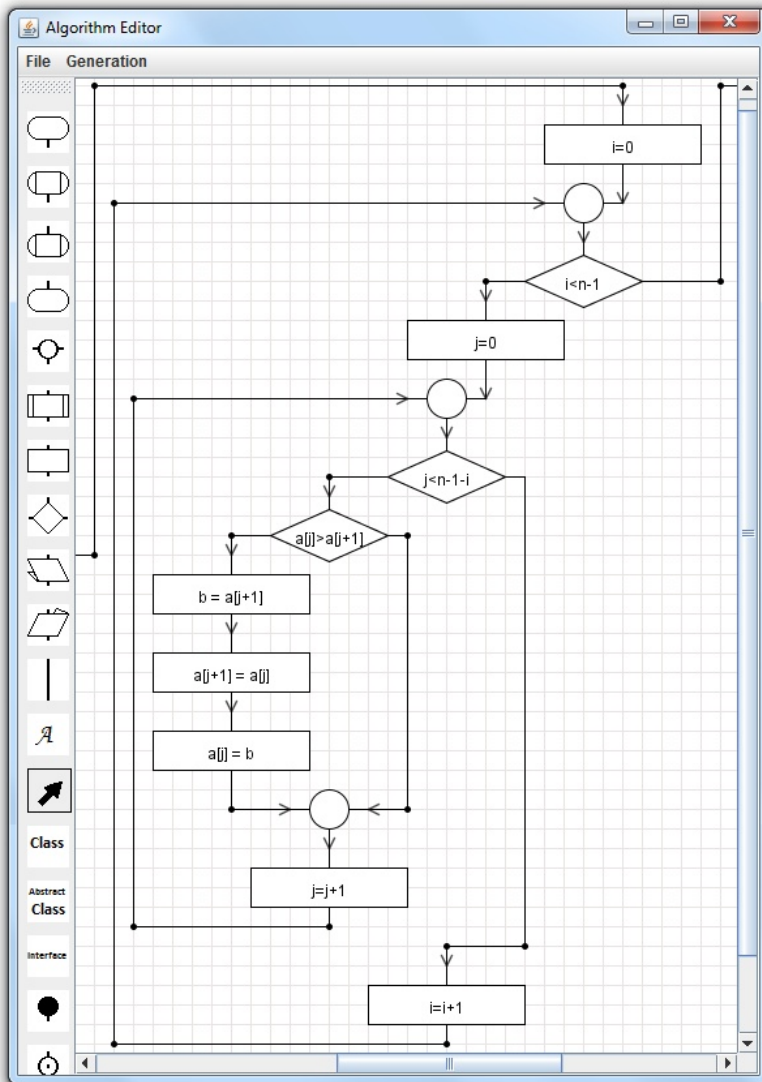
Рис. 1. Главное окно системы генерации с ГСА сортировки простыми обмени ("пузырьком")
